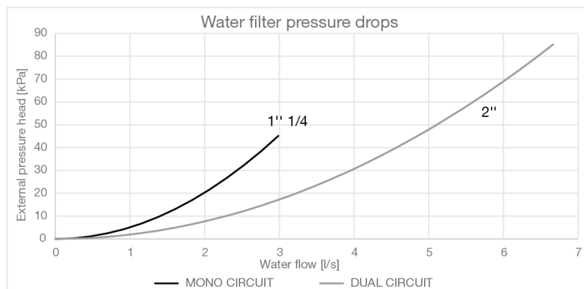
Afbeelding 17 – Drukverliezen waterfilter
