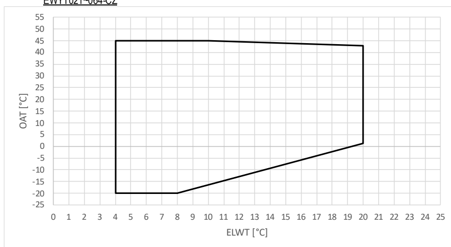
WERKINGSBEREIK KOELING- EWYT-CZ EWYT021-064-CZ
