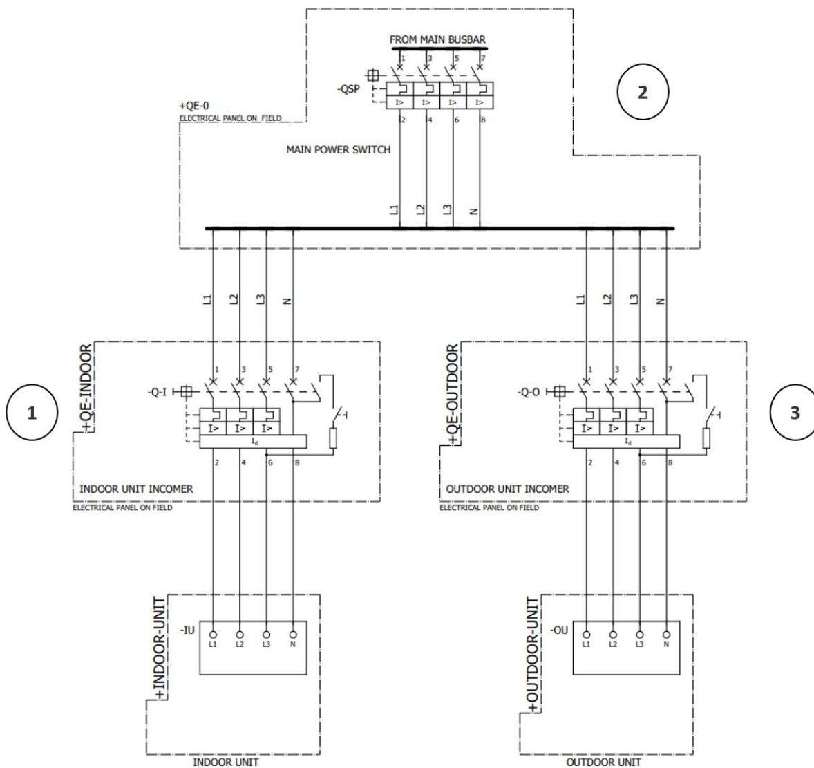
Afbeelding 20 – Master Bedradingsschema
