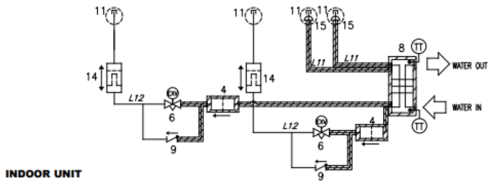
Afbeelding 25 – Koelcircuit (P&ID) schema voor DUAL-circuit EWYT~CZ-binnenunit
