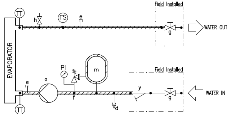
15. ábra – Hidraulikus diagram
