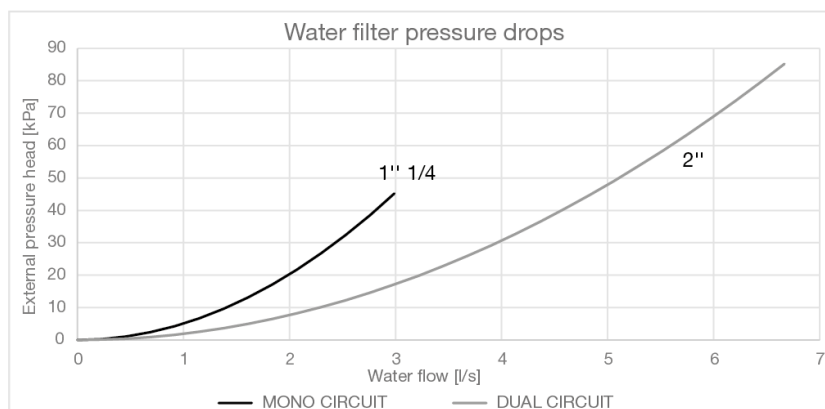
17. ábra – Vízszűrő nyomásesései
