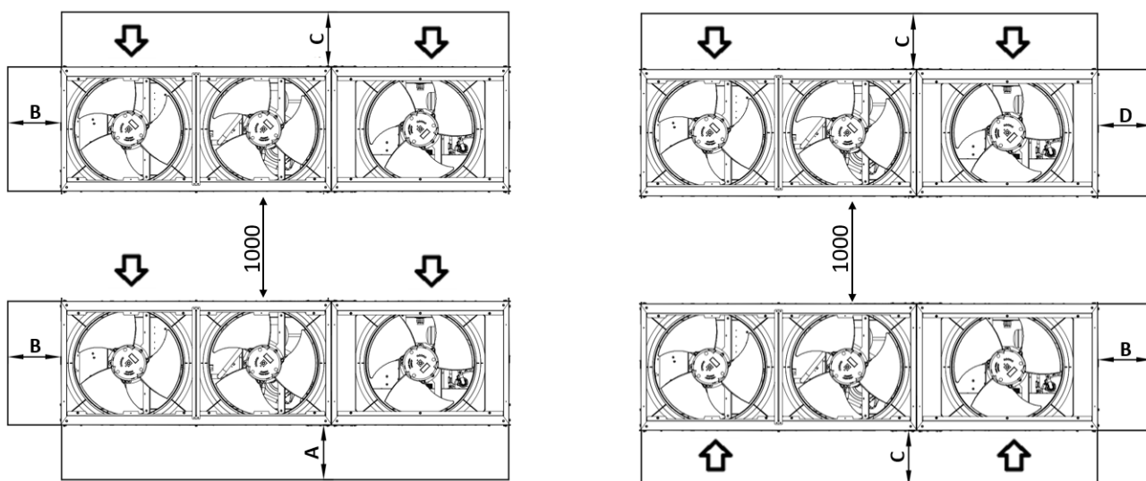
11. ábra – Hosszú oldaluk (1. vagy 2. példa) mentén egymás mellé telepített egységek
