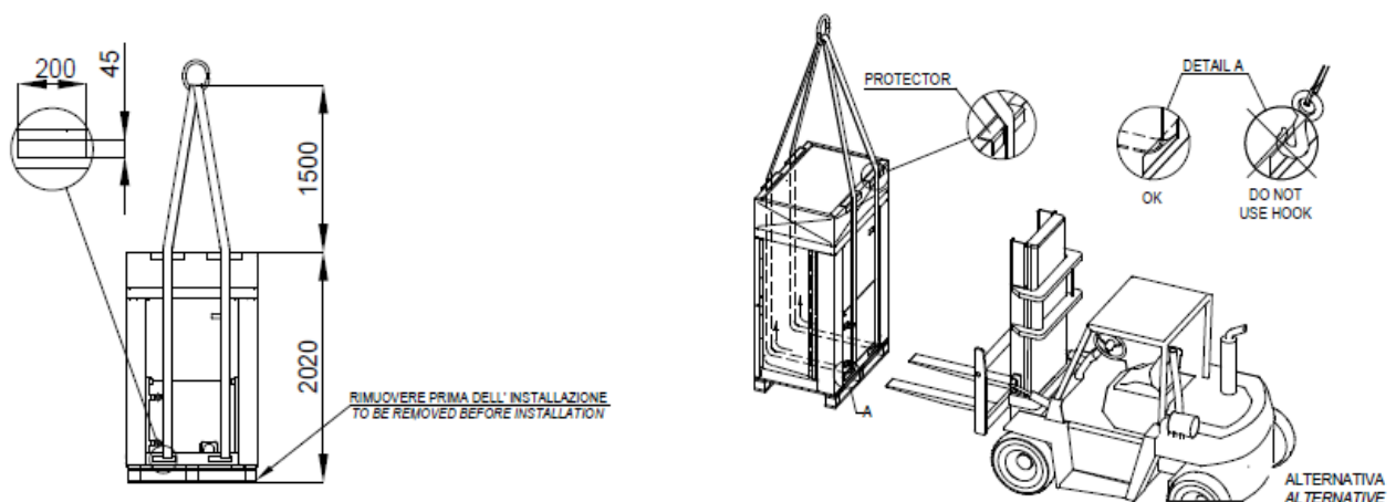
Obrázek 3 – Zvedání venkovní jednotky MONO
