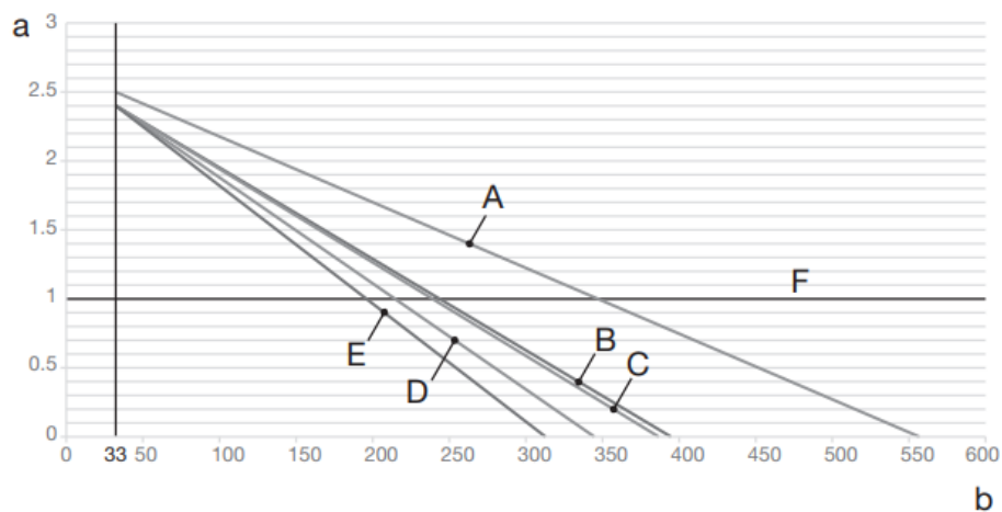
Рисунок 17 - Початковий тиск розширювального баку в залежності від максимального об'єму води
