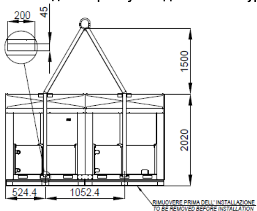
Рисунок 2 - Підйом агрегату з ПОДВІЙНИМ контуром
