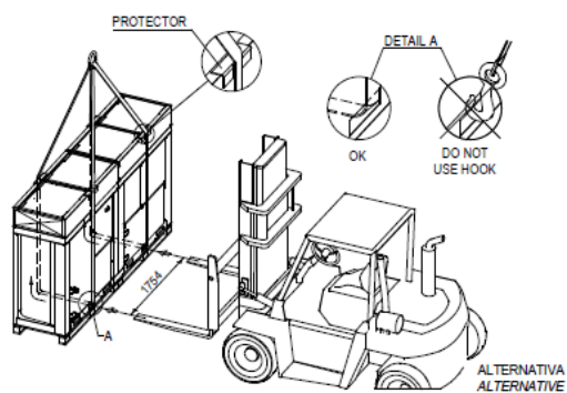
Рисунок 1 – Підйом агрегату з ОДНИМ контуром
