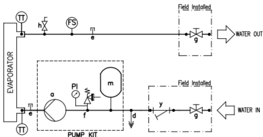
Рисунок 10 -Гідравлічна схема
