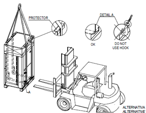
Рисунок 1 – Підйом агрегату з ОДНИМ контуром
