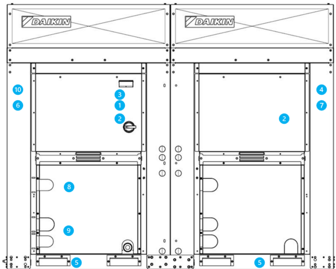
Рис. 22 - Наклейки на агрегате
