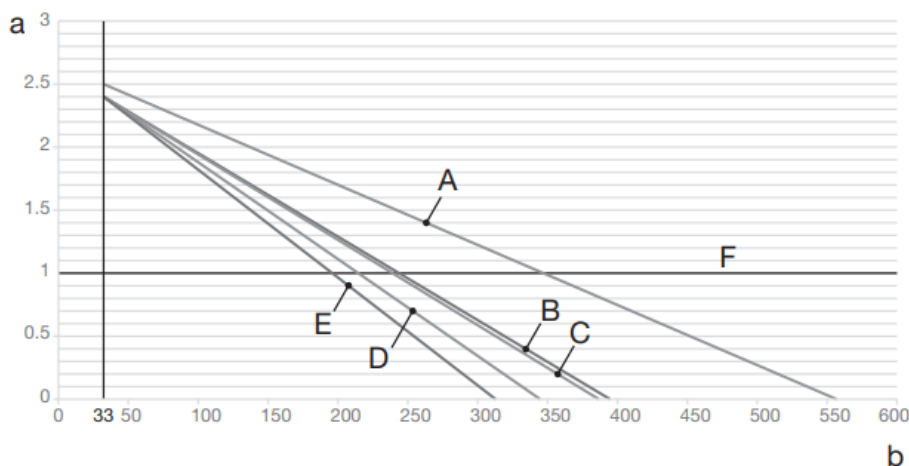
Рис. 17 - Начальное давление в расширительном баке на основе максимального объема воды
