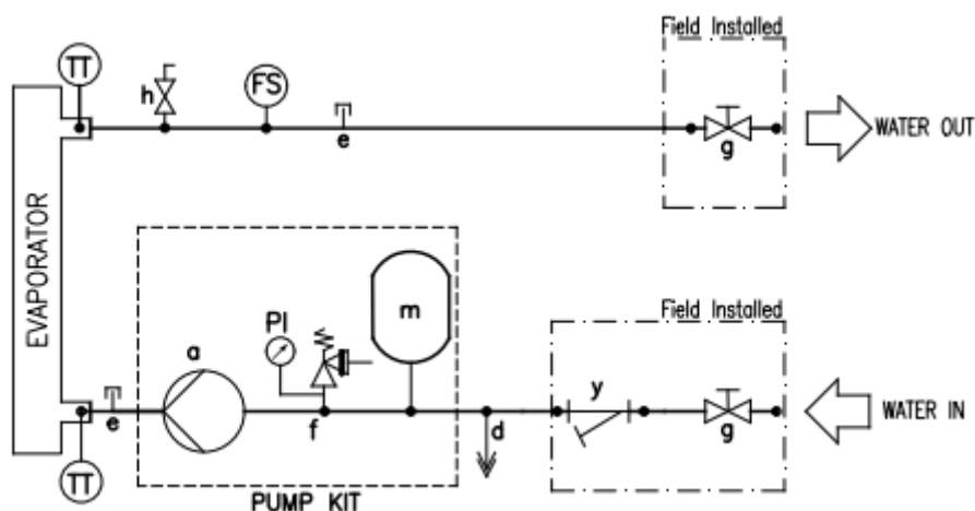
SI. 10 – Hidraulički dijagrami
