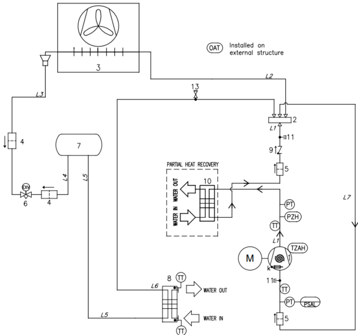
Εικόνα 18 - Διάγραμμα κυκλώματος ψυκτικού μέσου (P&ID) για μονάδα MONOY κυκλώματος EWYT~CZ
