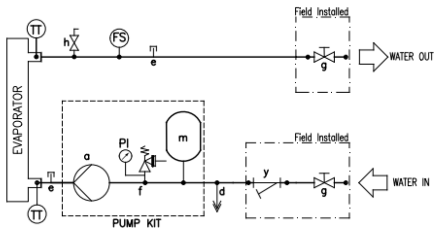
Figura 10 –Schema hidraulică
