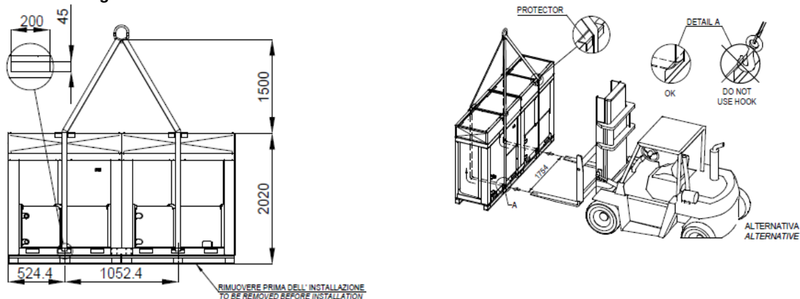
Figura 2 –Sollevamento dell'unità DUAL
