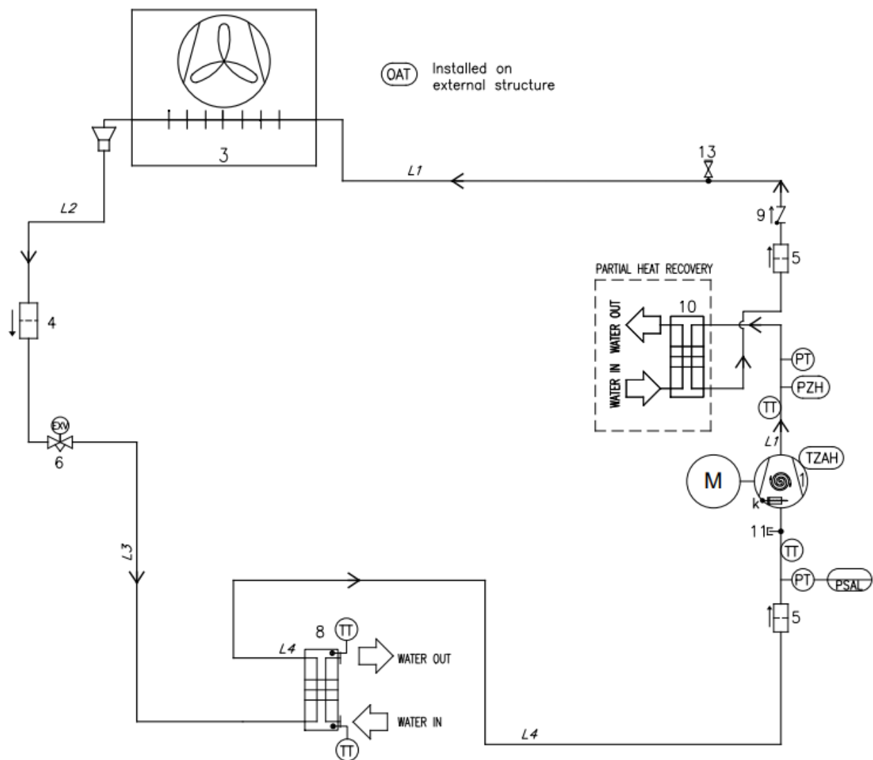
Abbildung 19 - Kältemittel (P&ID)-Kreislaufschemata für MONO-Kreislauf EWAT-CZ-Gerät
