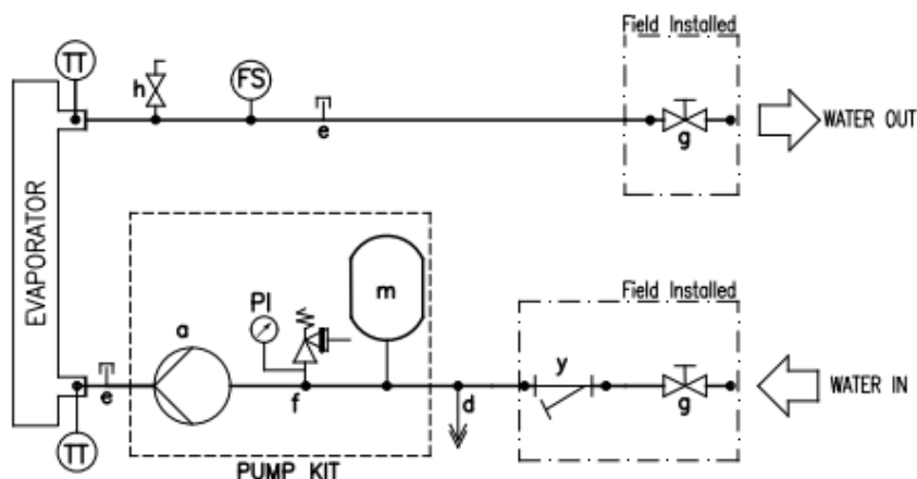
Obrázek 10 – Hydraulické schéma
