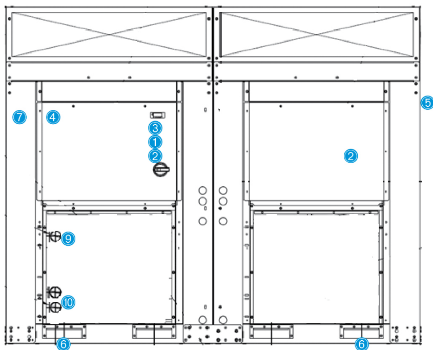
Obrázek 22 - Štítky na jednotce
