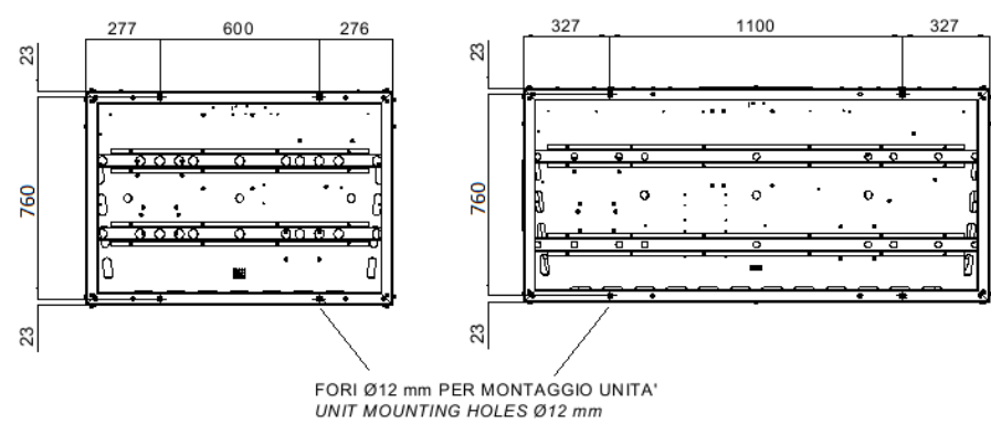
DISPOSIZIONE FORI MONTAGGIO (VISTA DAL BASSO) MOUNTING HOLES LOCATION (BOTTOM VIEW)
