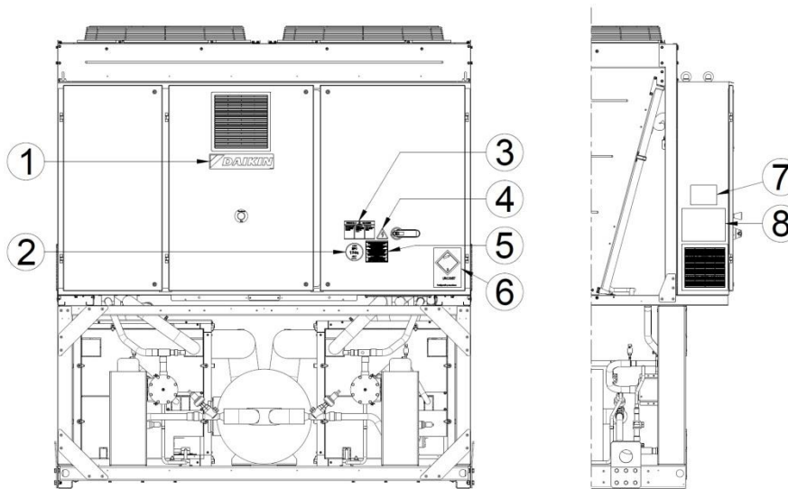
Unitate cu circuite duble
