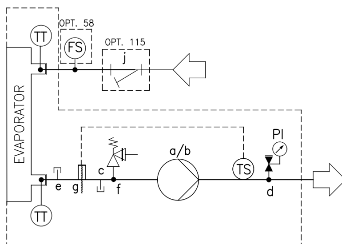
Fig. 7 - Raccord de tuyauterie d'eau
