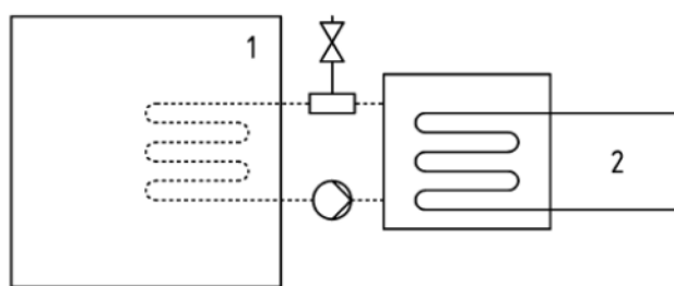
Systeme fermé à évacuation indirecte
