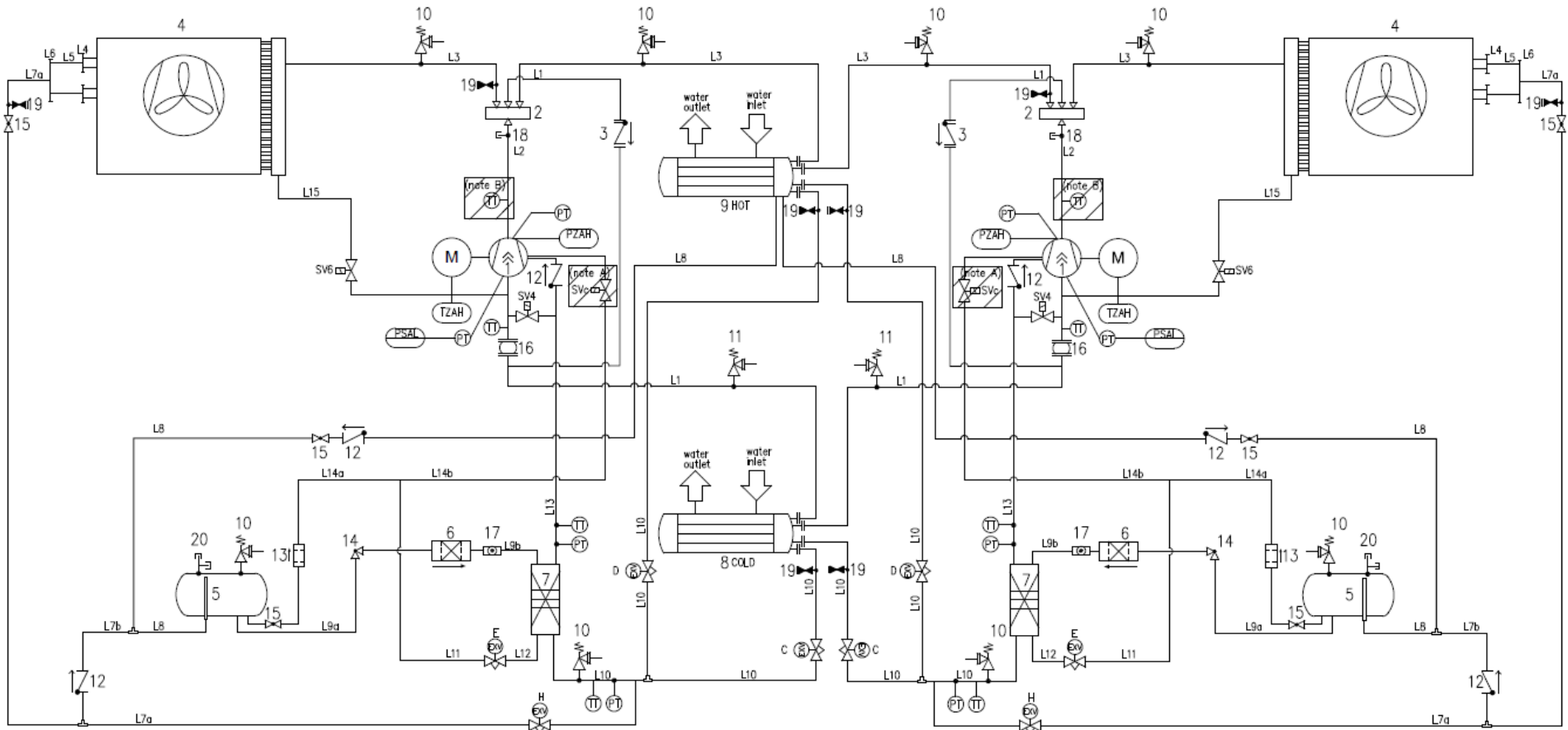
Fig. 1 - EWYD-4Z / EWYS-4Z Circuito de refrigerante típico
