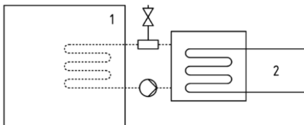
Fig. 18- Indirekt ventilerat slutet system
