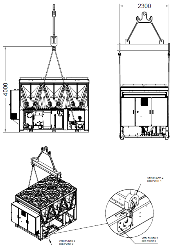
Enhet med fyra lyftpunkter
