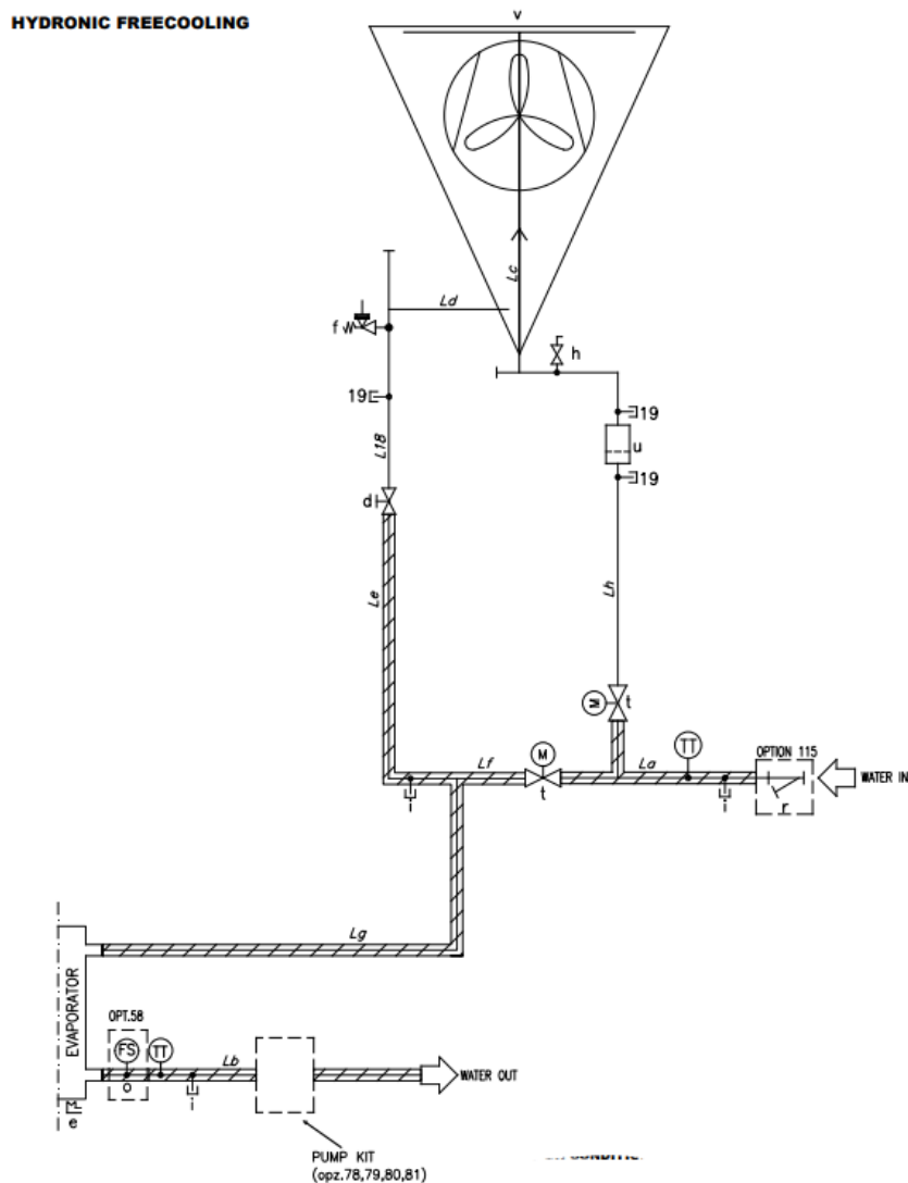
Fig. 27– Hydronisk frikylning P&ID
