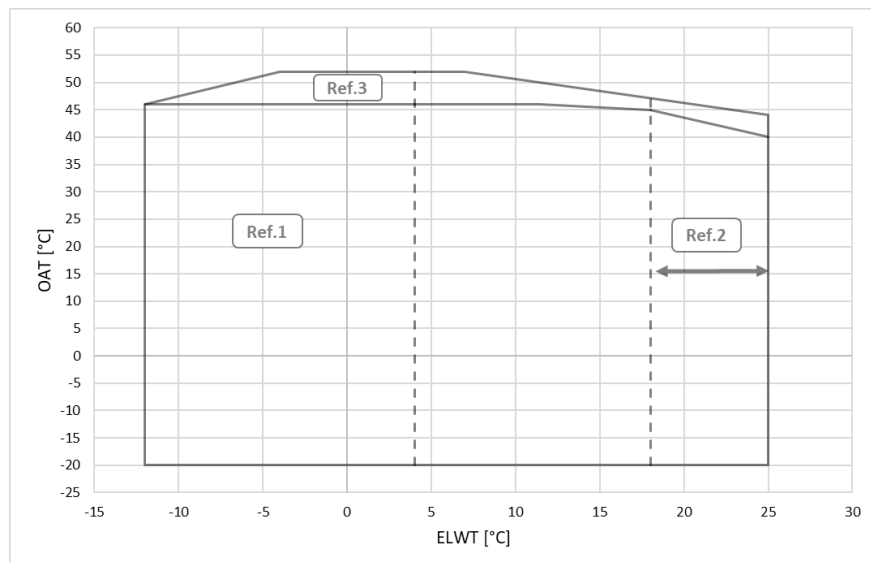
Fig. 17– EWFD-TZD guld och platina enhets område
