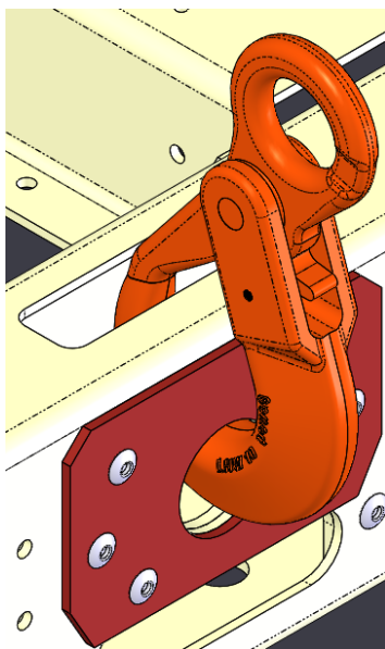
Fig. 20- Fästning av säkerhetskrok
