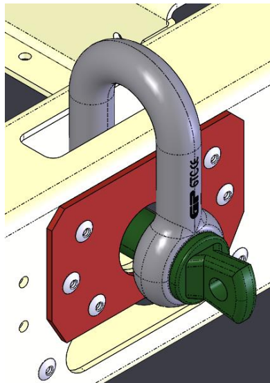
Fig. 21 Infästning av lyftsacklar
