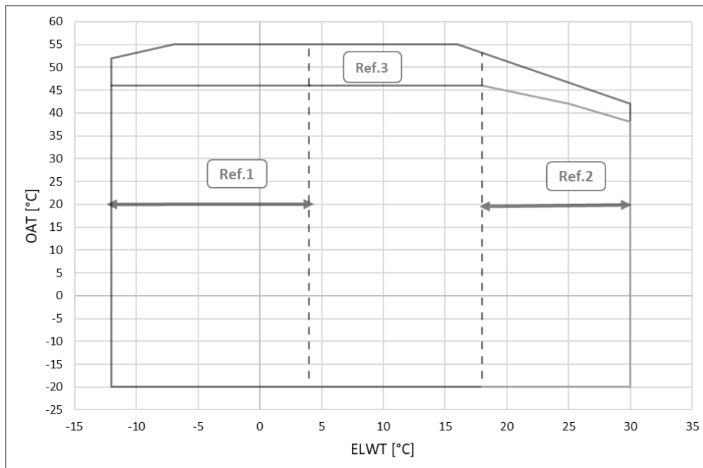
Fig. 15– EFFFH-TZD guld och platina enhets område
