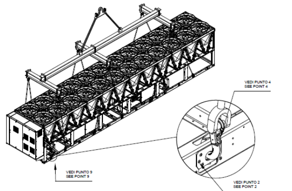
Fig. 19- Lyftanvisningar
