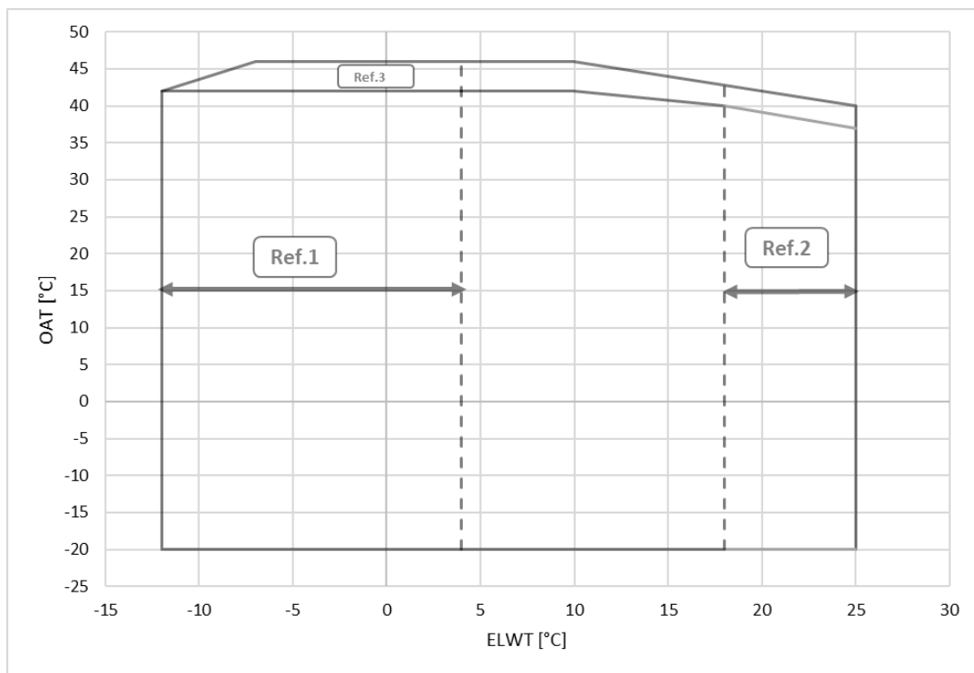
Fig. 13– EWAS-TZD guld och platina enhets område
