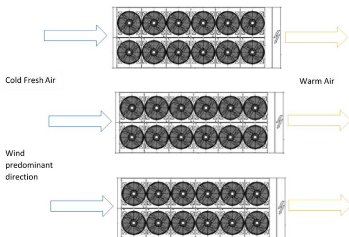
Fig. 25– Installation av flera kylaggregat
