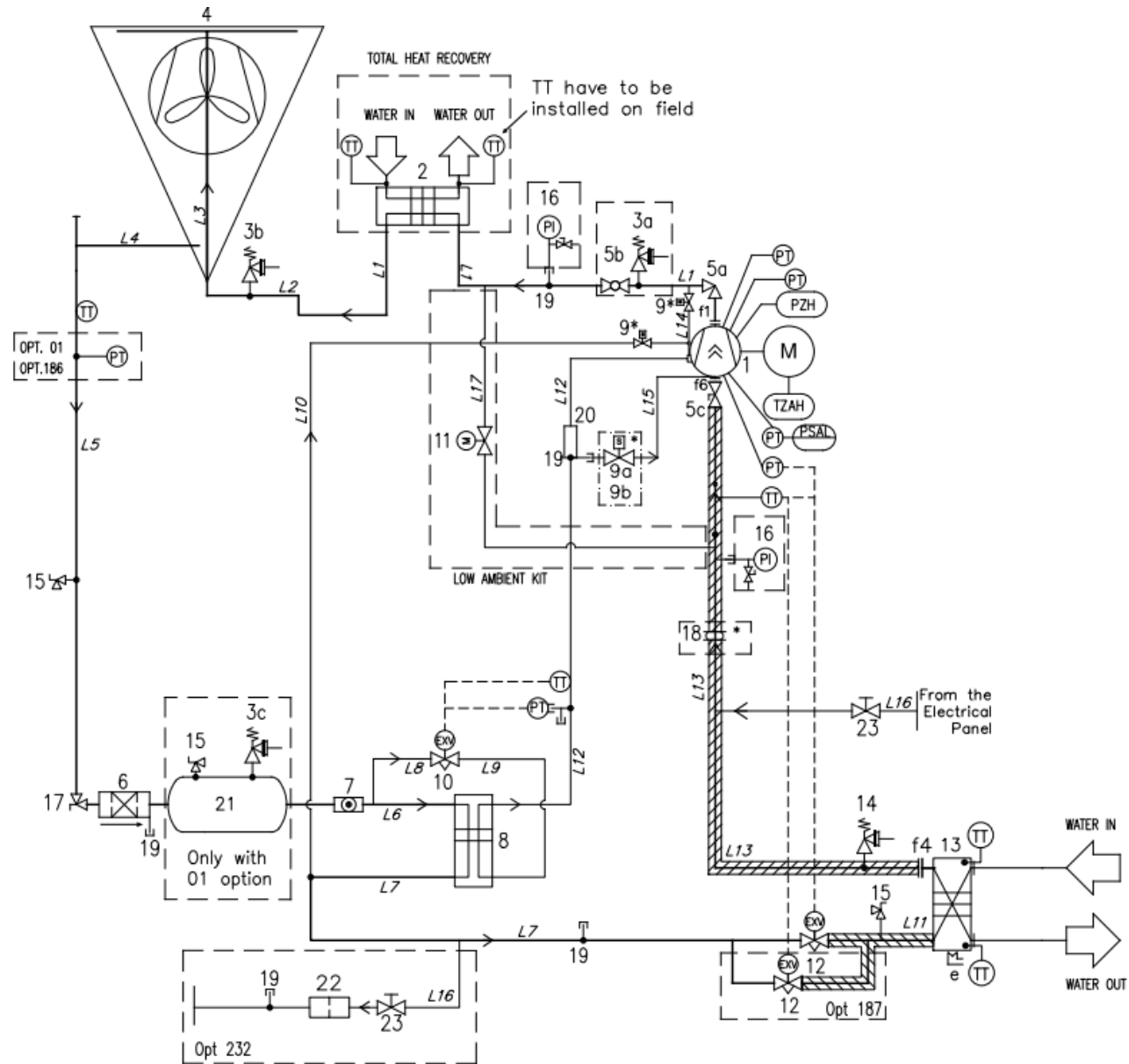
Fig. 1- Kylmedelskrettschema (P&ID) – MONO kretsener
