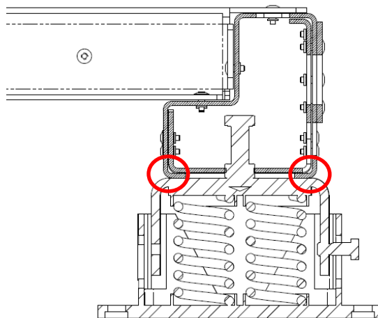
Fig. 23- Montering av vibrationsdämpande element (levereras som tillval)
