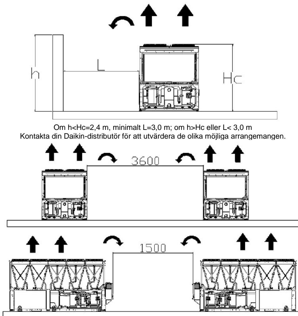
Fig. 24- Minimikrav för fri höjd
