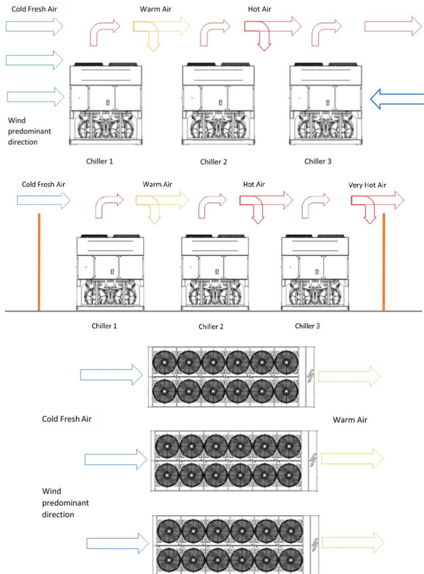
Fig. 25. – Instalação de refrigerador múltiplo
