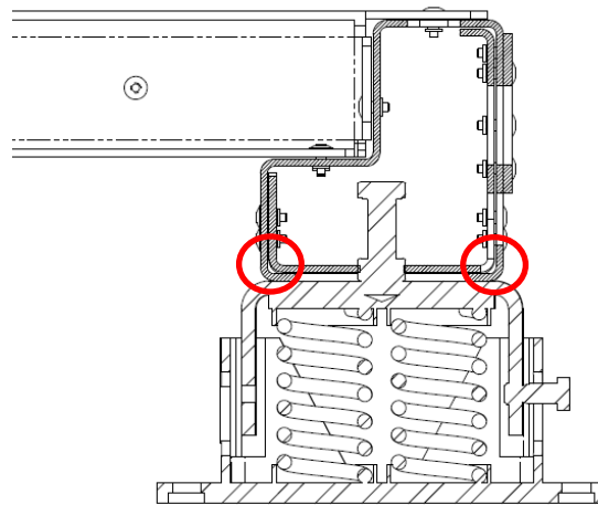
Fig. 23– Elementos antivibração de montagem (fornecidos como opcional)
