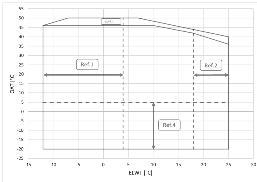
Fig. 8- Envelope da unidade EWAD-TZD Blue
