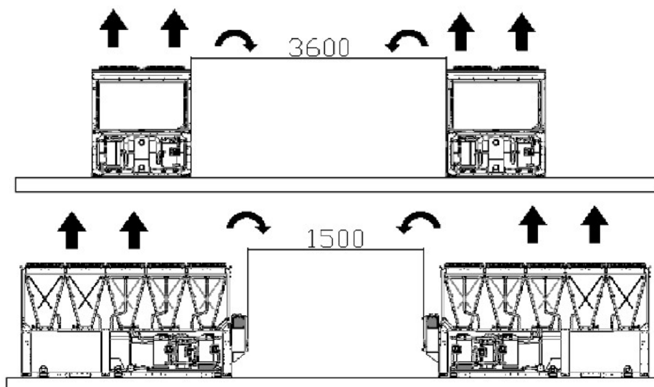
Fig. 24- Requisitos de mínimos espaços
