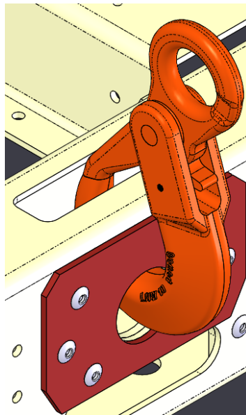
Fig. 20- Fixação do gancho de segurança
