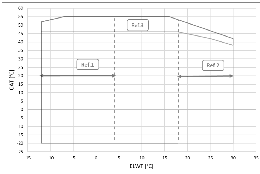
Fig. 15– Envelope da unidade EFWH-TZD Gold e Platinum
