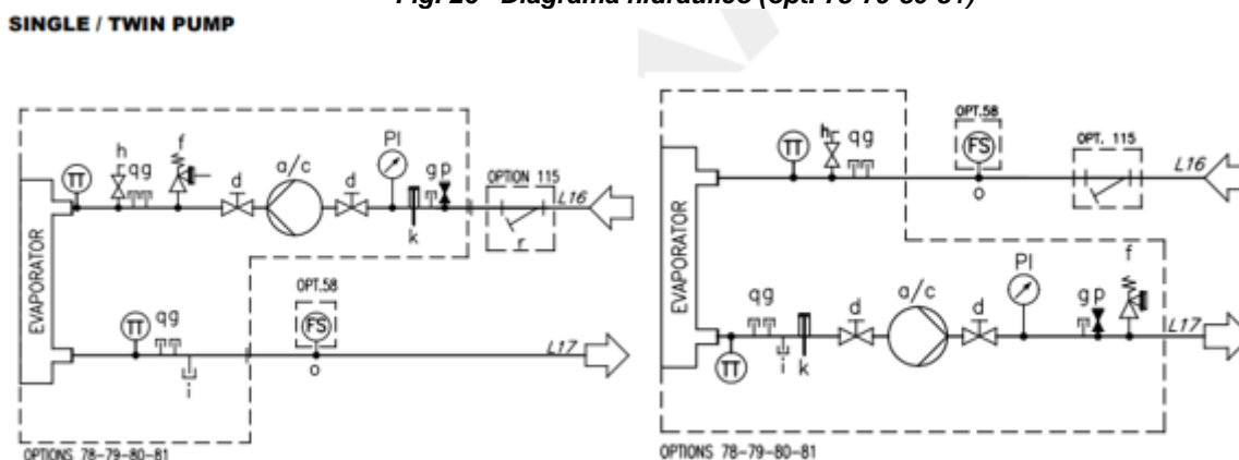
Fig. 26– Diagrama hidráulico (opt. 78-79-80-81)
