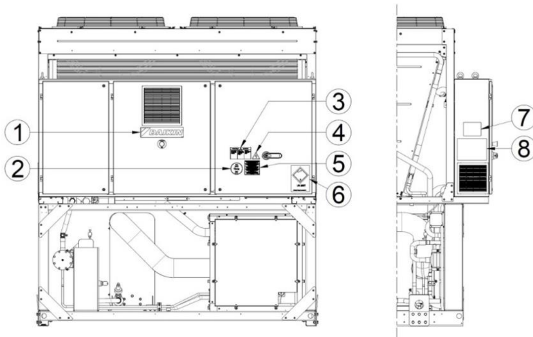
Fig. 4. - Descrição das etiquetas aplicadas ao painel elétrico
