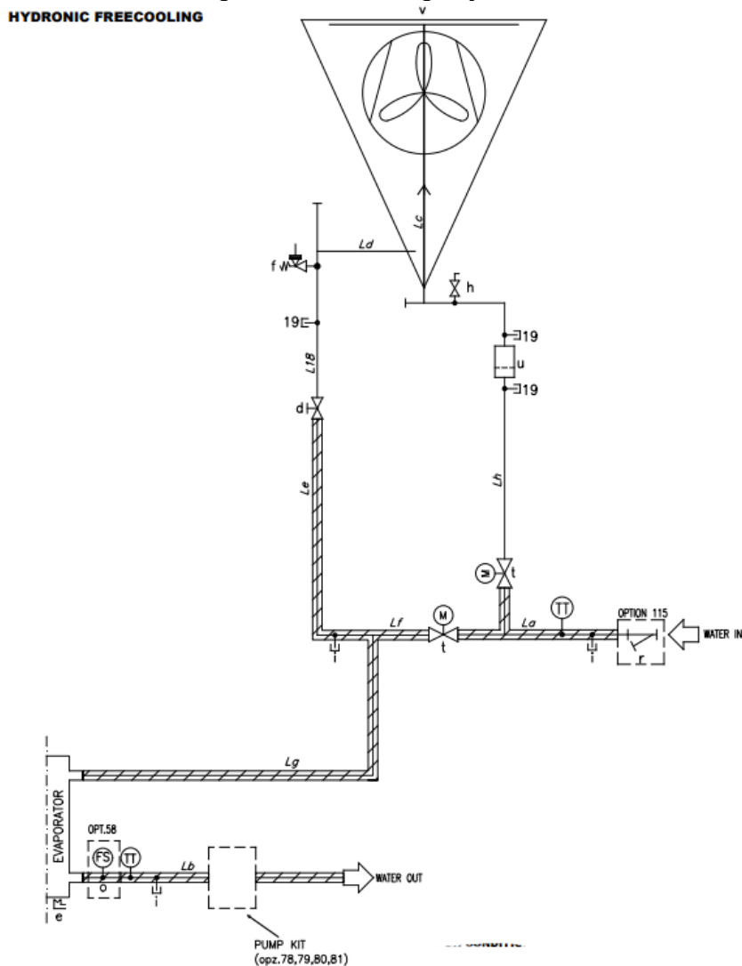
Fig. 27– P&ID de Refrigeração Livre Hidrónica
