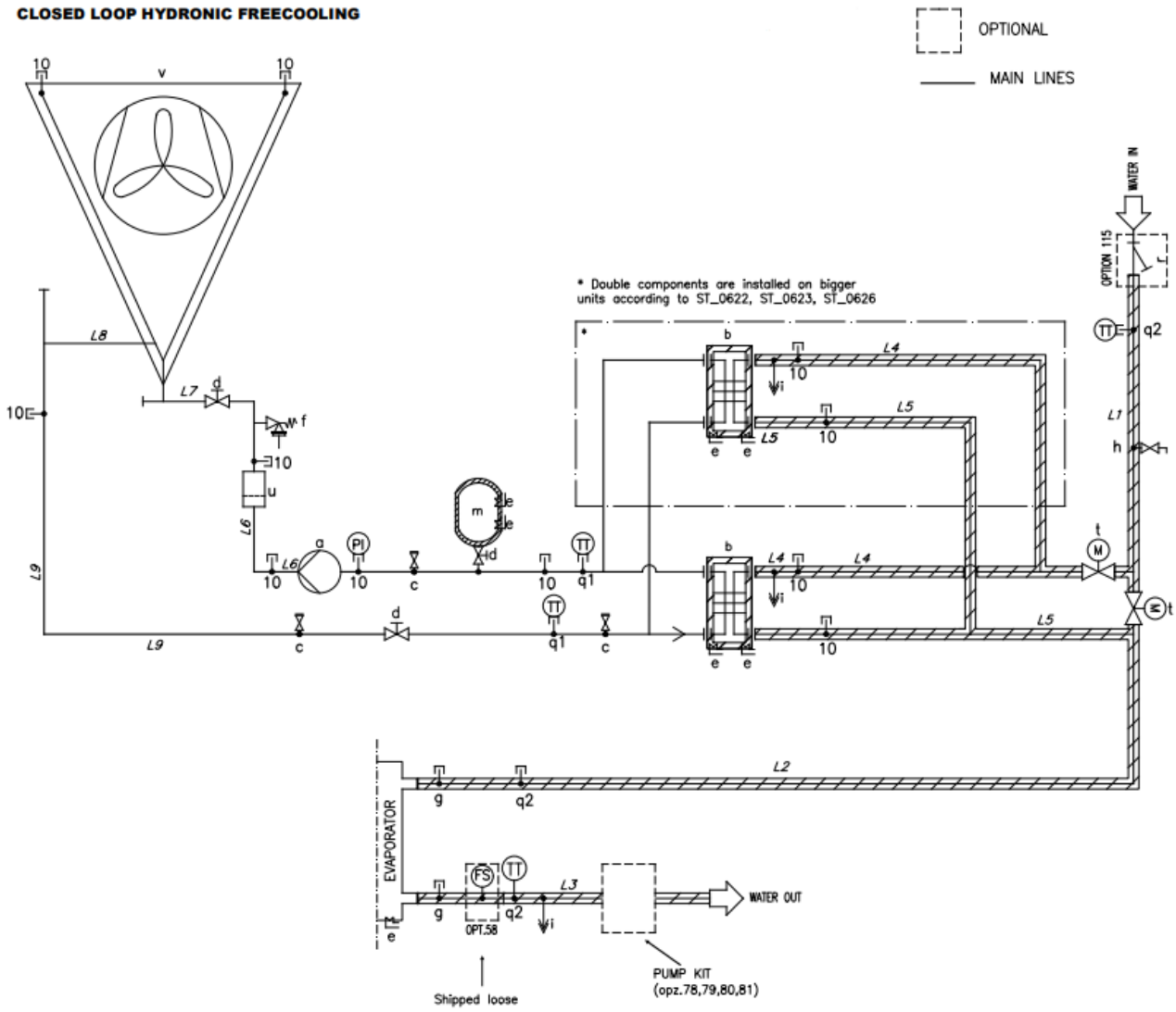
Fig. 3- Hydronische vrije koeling met gesloten circuit P&ID (Opt. 231)
