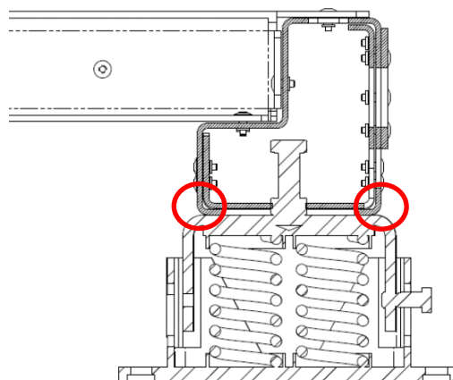
Afb. 21 – Antitrilelementen montage (geleverd als optie)
