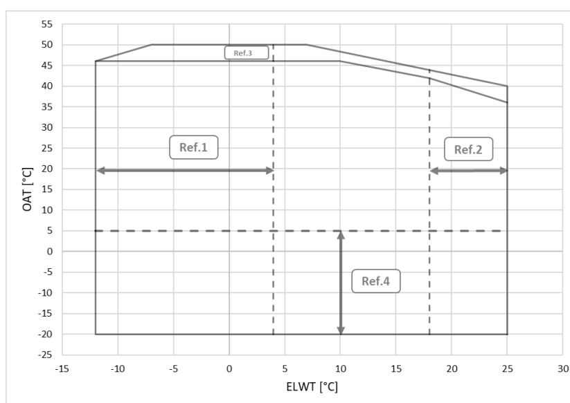
Afb. 8 – EWAD-TZD Blauwe eenhedvelop
