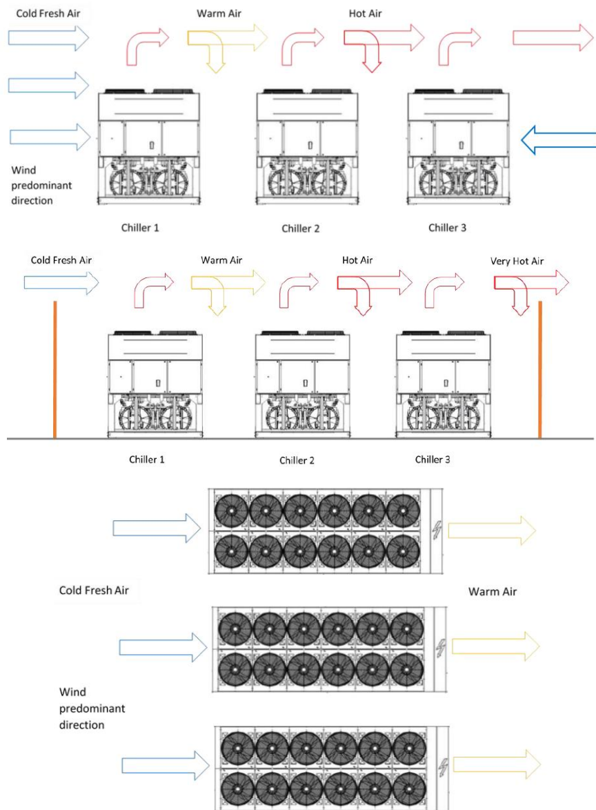
Afb. 23 – Installatie meerdere koelers
