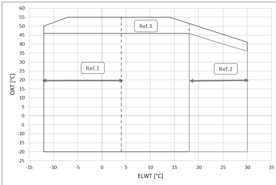
Afb. 14 – EFWH-TZD Blauwe en zilveren envelop
