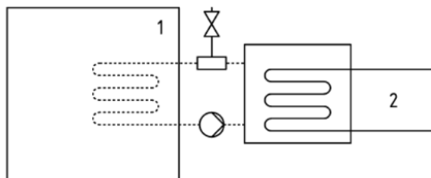
Afb. 18 - Indirect geventileerd gesloten systeem
