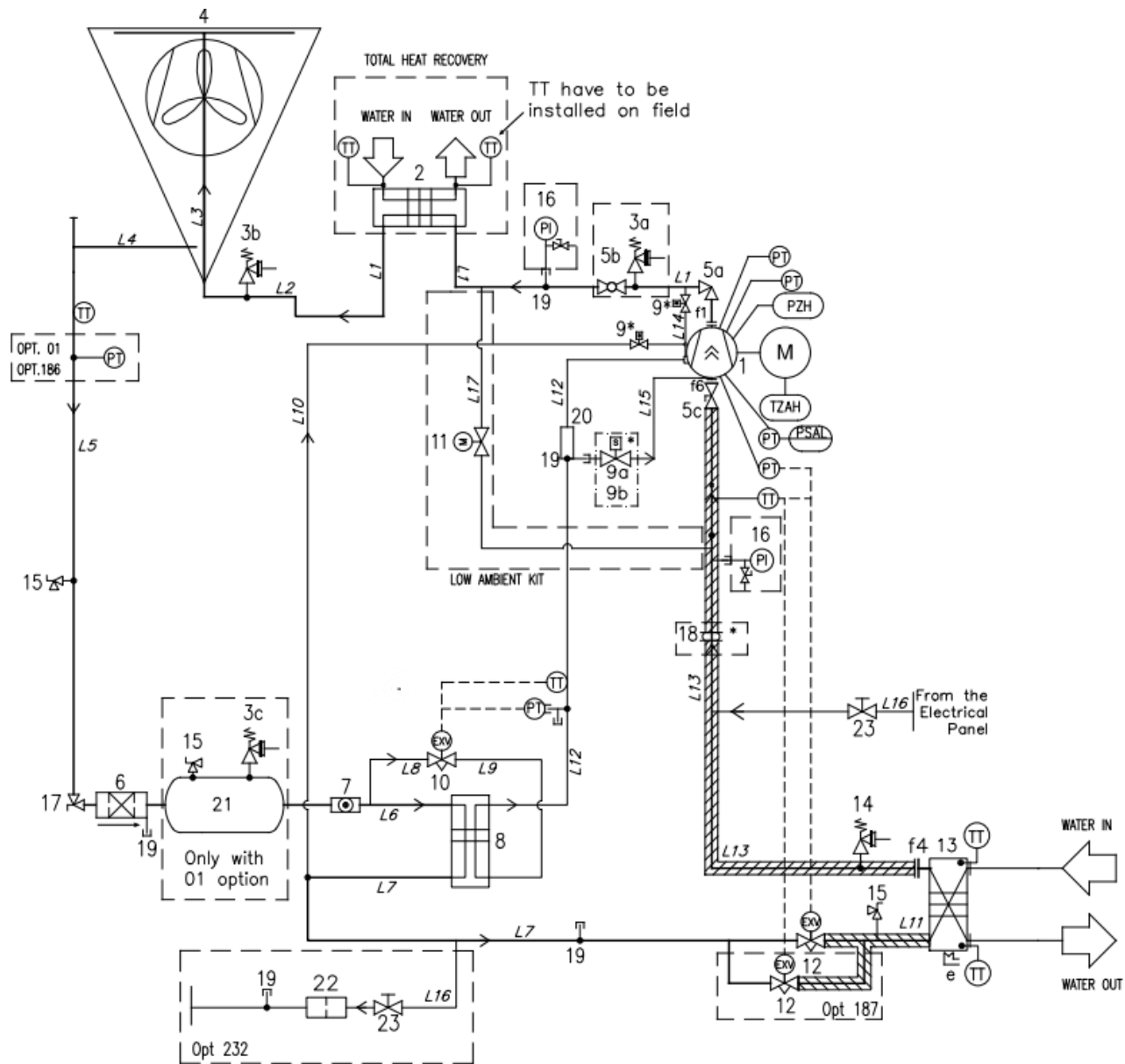
Afb. 1- Schema koelcircuit (P&ID) standaardstelsel met enkel circuit
