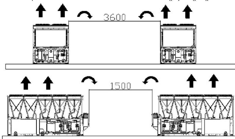
Afb. 22 - Minimaal vereiste afstanden
