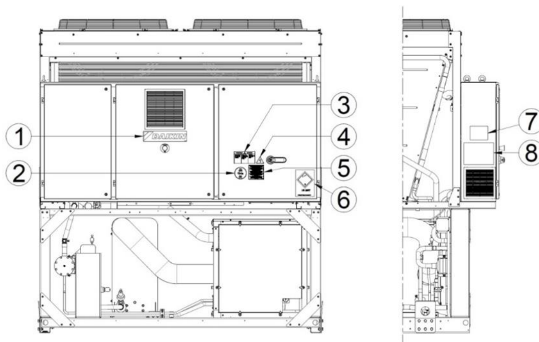
Εικ. 4 . - Περιγραφή των ετικετών που υπάρχουν στον ηλεκτρικό πίνακα
