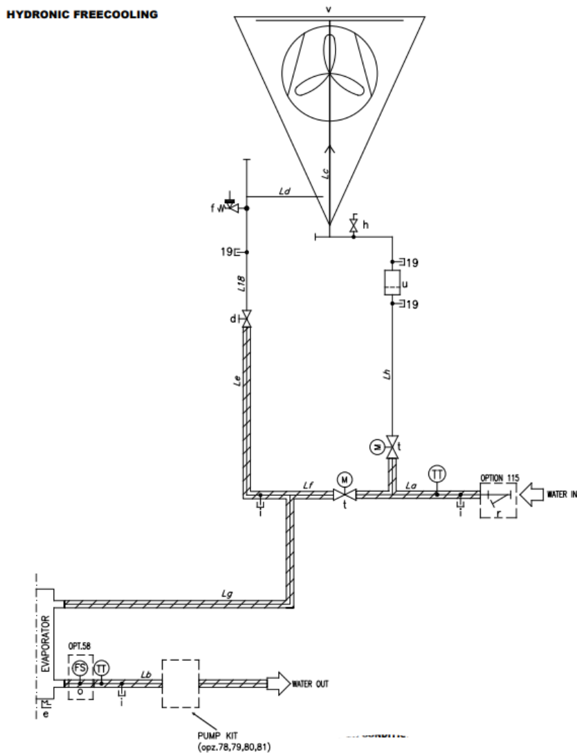
Εικ. 27 – Υδρονικό ελεύθερης ψύξης Διάγραμμα σωληνώσεων και οργάνων
