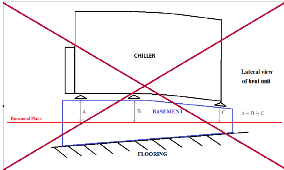
Εικ. 20 – Οριζοντίωση μονάδας
