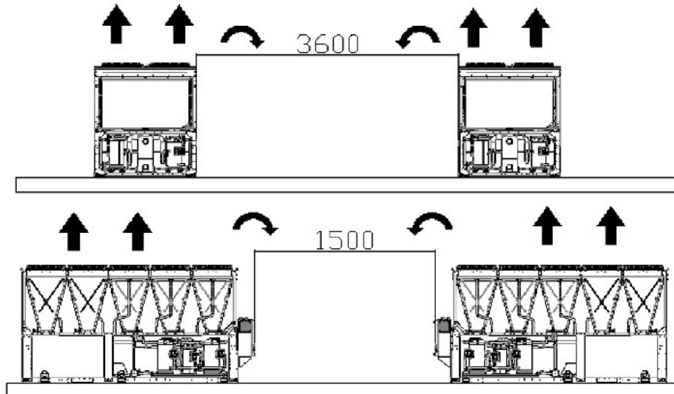
Εικ. 24 - Ελάχιστες απαιτήσεις χώρου
