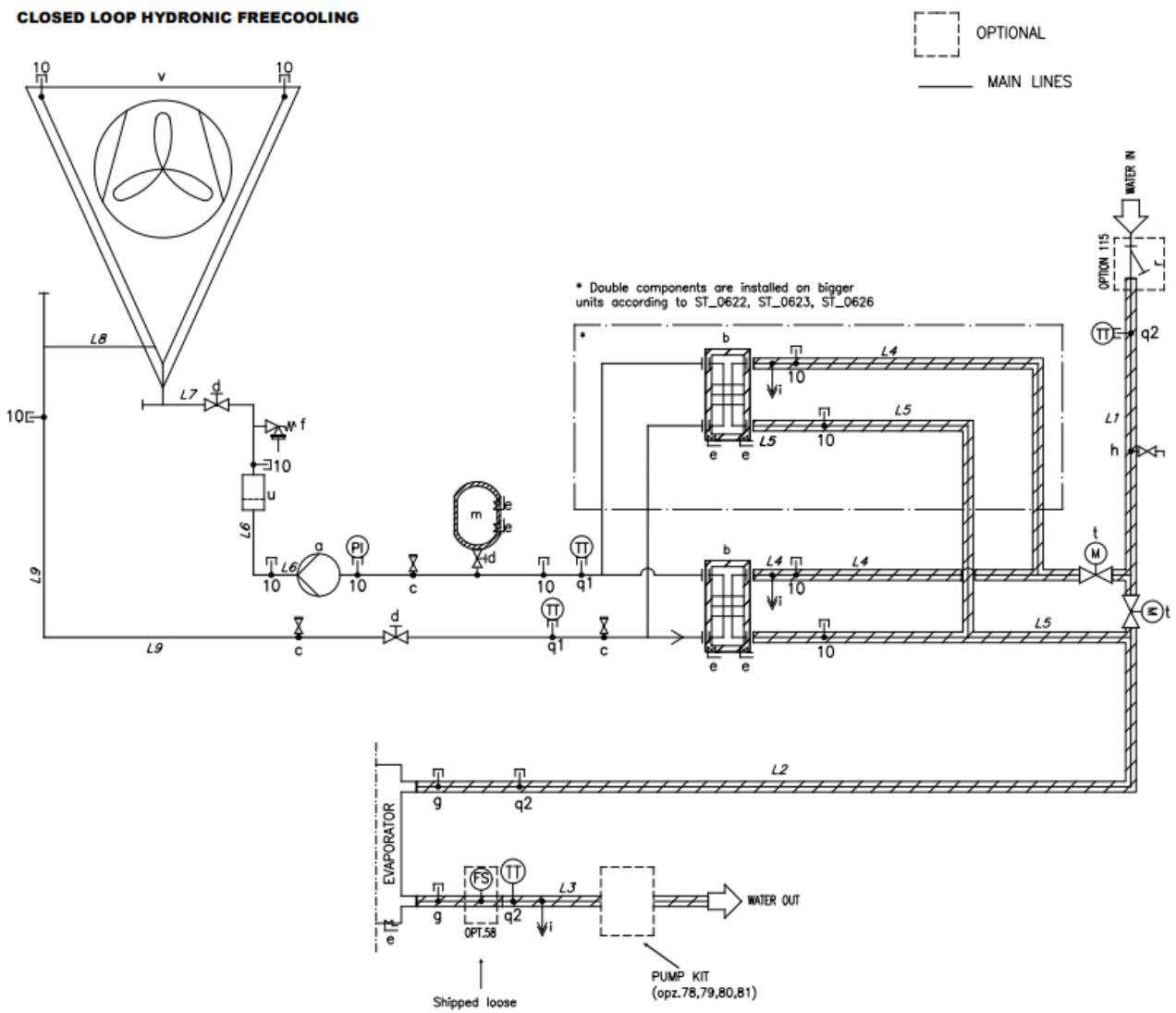
Εικ. 28 - Κλειστό κύκλωμα υδραυλικής ελεύθερης ψύξης P&ID (Opt. 231)
