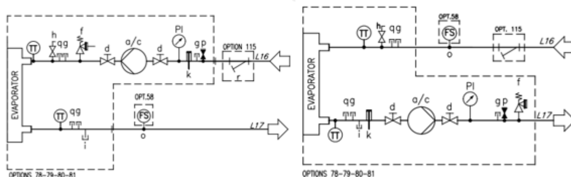
Πίνακας 12 –Υπόμνημα Διάγραμμα υδραυλικού
