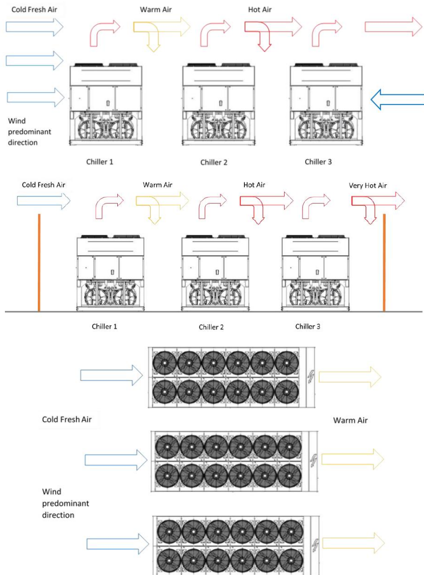
Εικ. 25 – Εγκατάσταση πολλών ψυκτών
