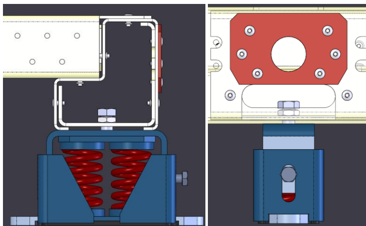
Sl. 21– Konačna pozicija antivibracionog prigušivača.
