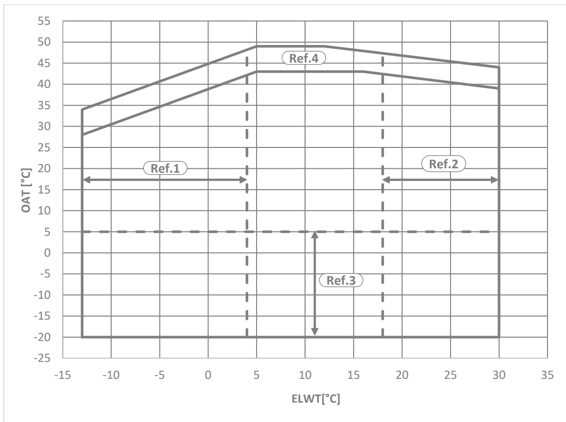
Sl. 4 Ograničenja rada za EWAT-B-C Silver
