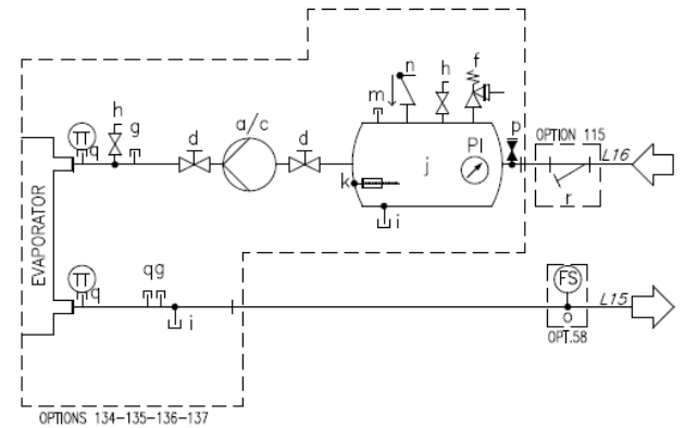
Sl. 22- Hidraulički dijagram (opc. 78-79-80-81/134-135-136-137)
