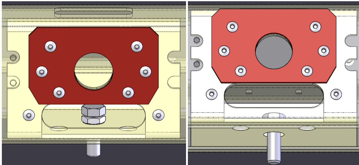
Sl. 19–Detalj zavrtnja za pričvršćivanje amortizera protiv vibracija
