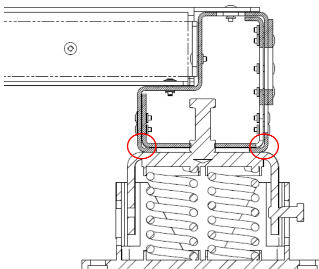
SI. 18 - Montaža antivibracionih elemenata (isporučuju se kao opciono delovi)
