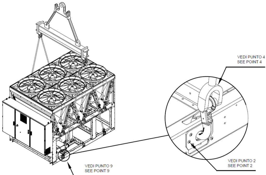
Jedinica sa 4 tačke za podizanje Crtež prikazuje samo verziju sa 6 ventilatora. Režim podizanja je isti bez obzira na broj ventilatora
