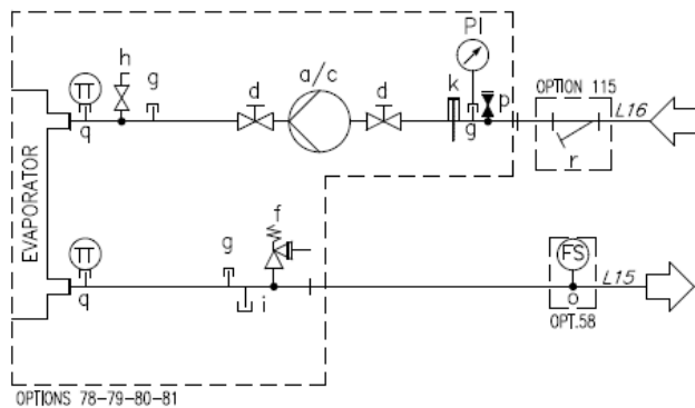
Sl. 22- Hidraulički dijagram (opc. 78-79-80-81/134-135-136-137)
