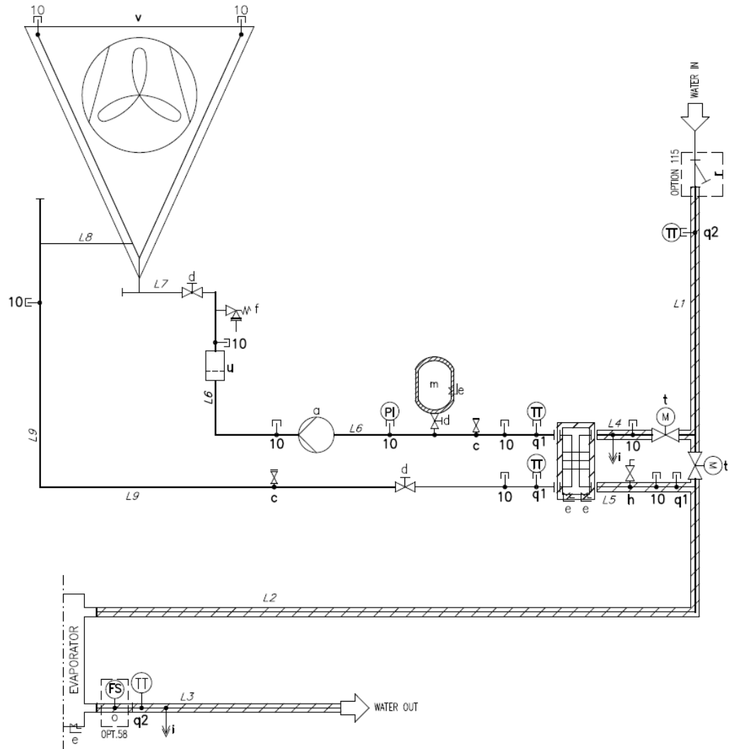
Sl. 24– Zatvorena petlja Hidronic P&ID za slobodno hlađenje (Opt. 231)
