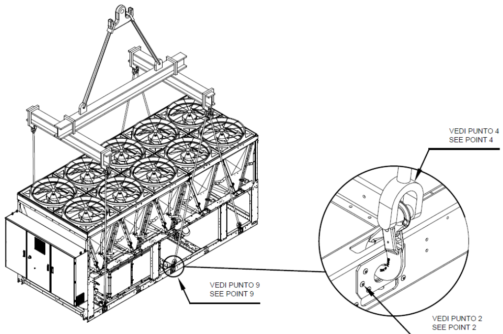
Jedinica sa 6 tačke za podizanje Crtež prikazuje samo verziju sa 10 ventilatora. Režim podizanja je isti bez obzira na broj ventilatora.
