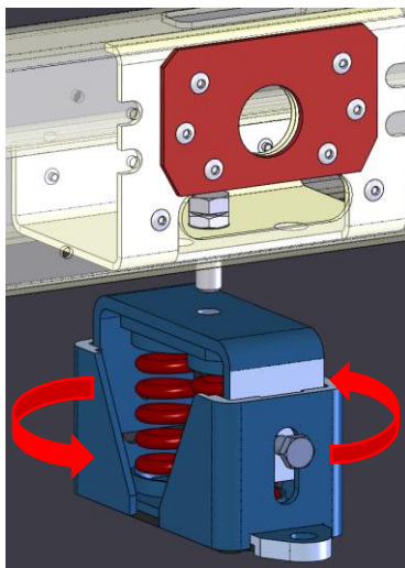
Sl. 20– Detalj ugradnje prigušivača protiv vibracija.
