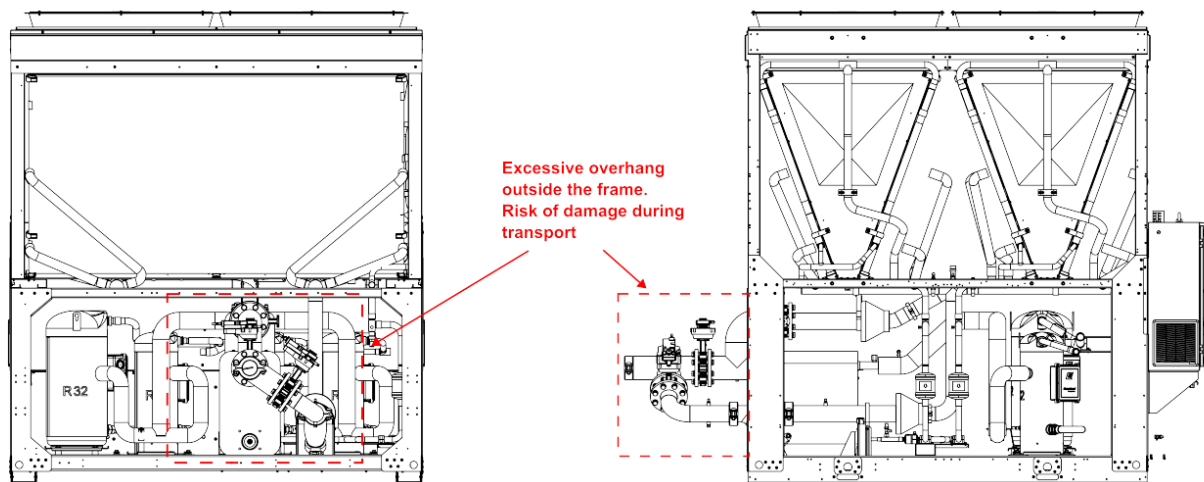
Sl. 16- Cevovodi izvan otiska jedinica za slobodno hlađenje.
