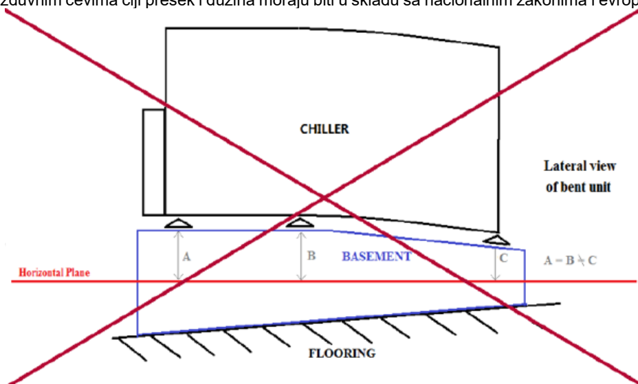
Sl. 13- Nivelisanje jedinice
