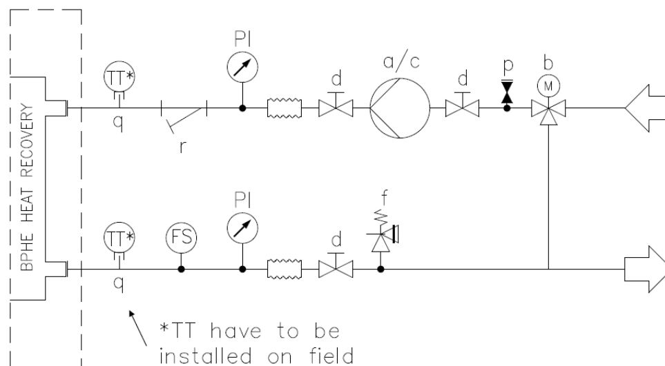
Sl. 23- Priključak vodovoda za izmenjivače sa rekuperacijom toplote (maksimalni pritisak od 20 bara)
