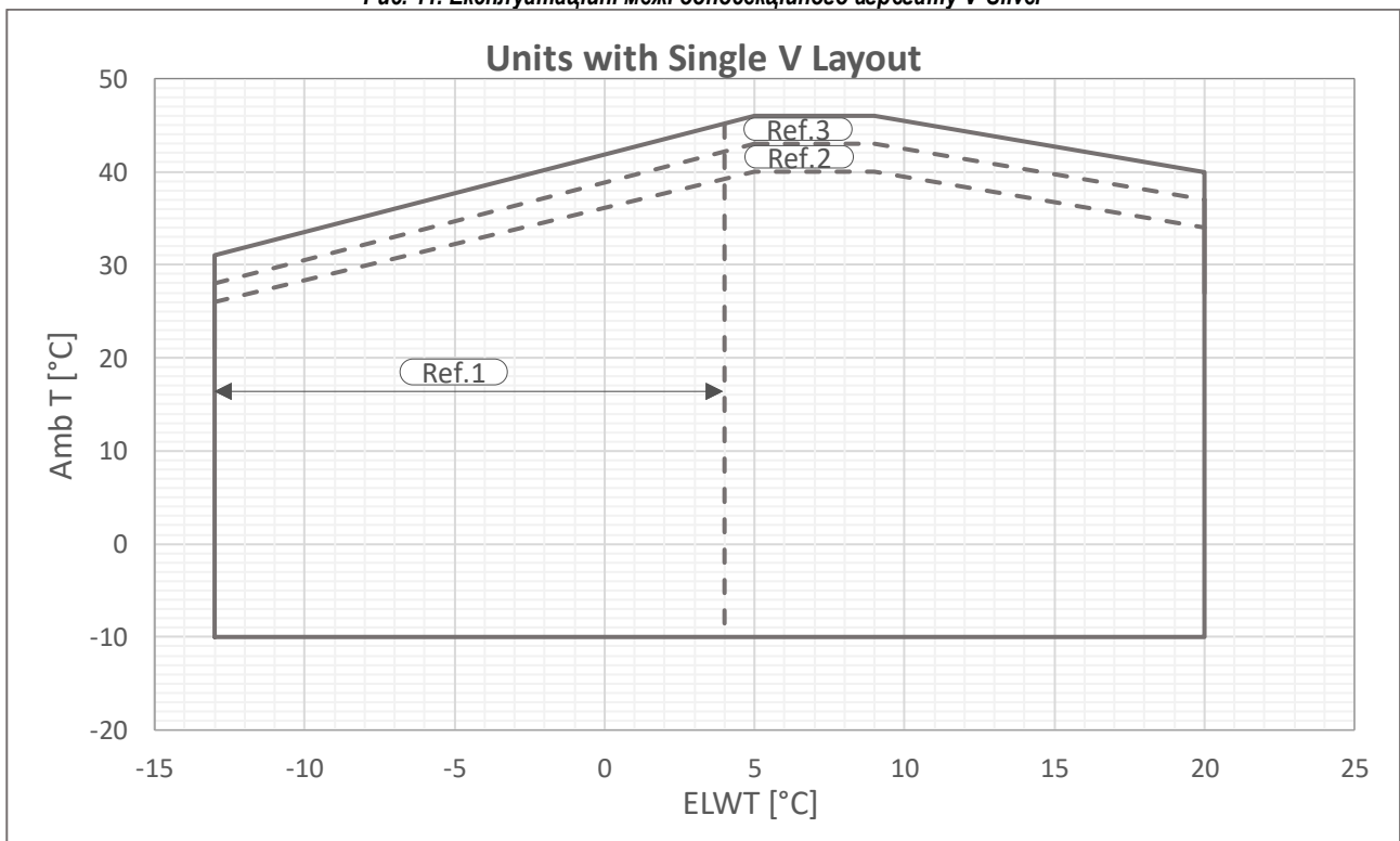
Рис. 12. Експлуатаційні межі односекційного агрегату V-Gold
