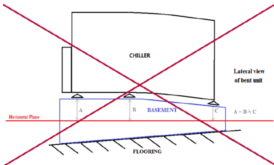
Рис. 2. Вирівнювання агрегату
