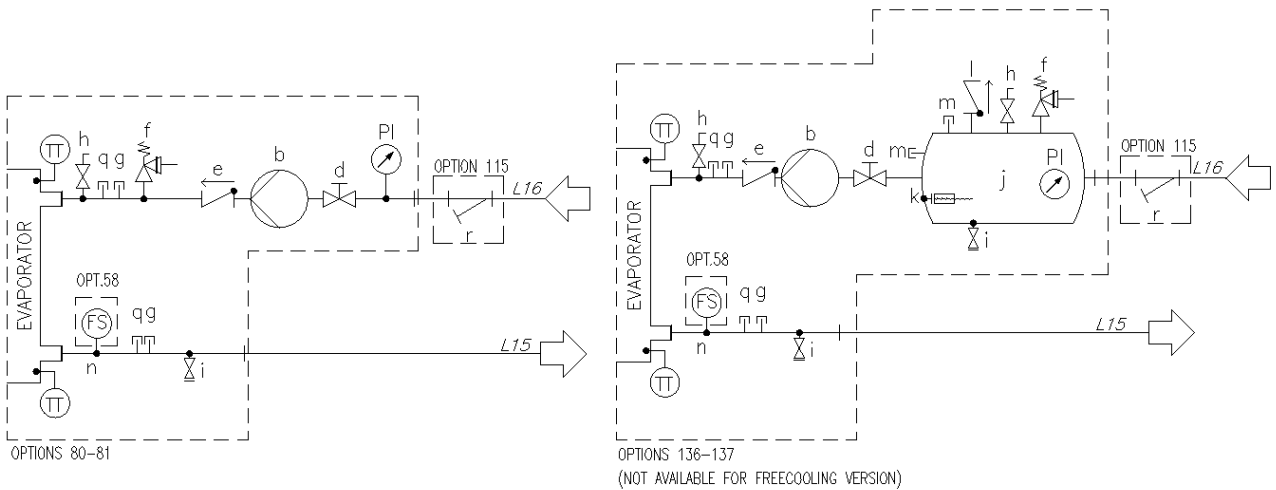
Рис. 7. Гідралічна схема односекційного агрегату (EWATxx5B) зі здовєним насосом (компл. 80-81/136-137) (макс. робочий тиск 6 бар)
