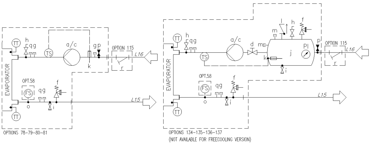
Рис. 8. Гідралічна схема мультисекційного агрегату (EWATxx0B) (компл. 78-79-80-81/134-135-136-137) (макс. робочий тиск 6 бар)
