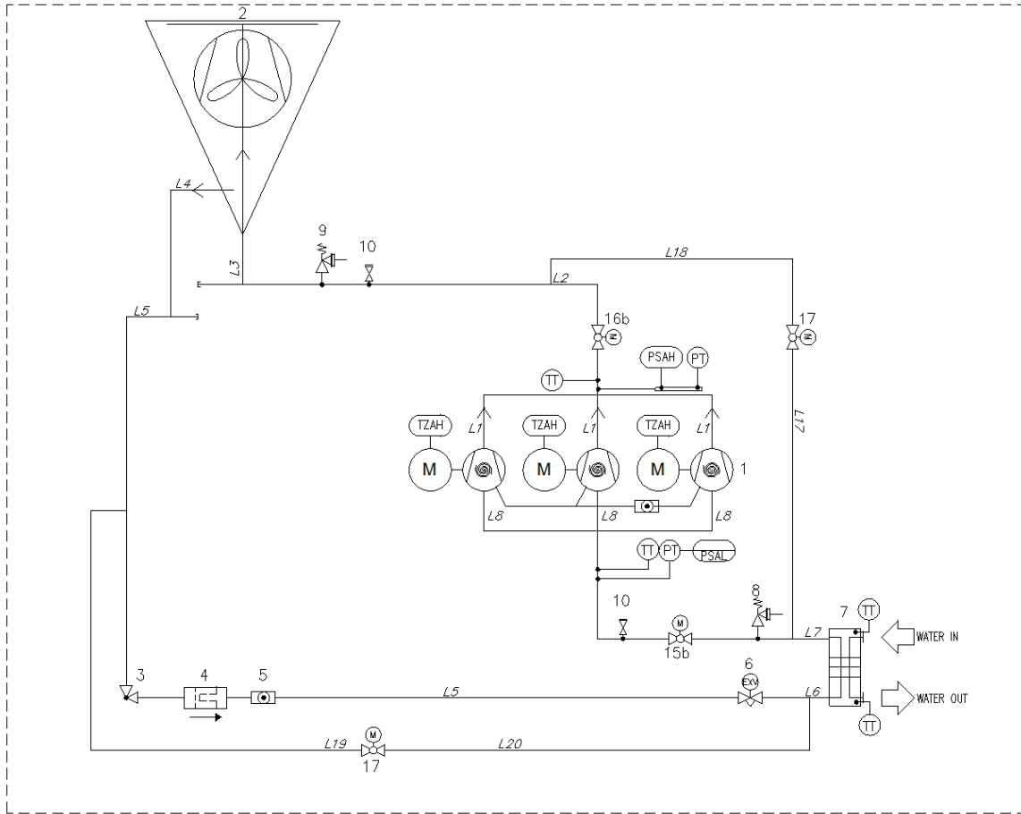
Рис. 14. Схема контуру холодоагенту (схема трубопроводів і КВП) для типового одноконтурного агрегату з частковим природним охолодженням
