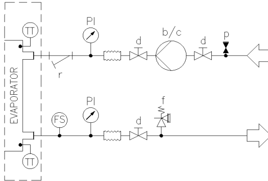
Şekil 5 – Cihazda pompa(lar) olmadan hidrolik diyagram (maks. çalışma basıncı 20 bar)
