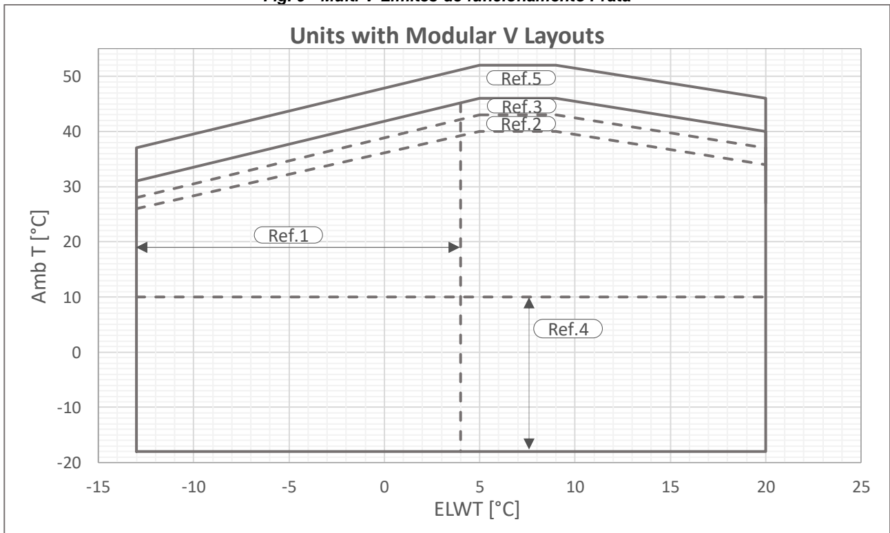
Fig. 10 - Multi V-Limites de funcionamento Ouro
