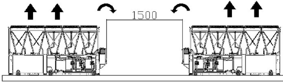
Fig. 3 - Requisitos mínimos de espaço
