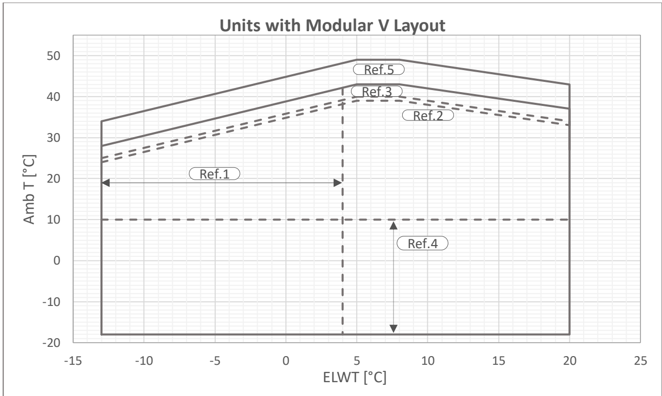
Fig. 9 - Multi V-Limites de funcionamento Prata
