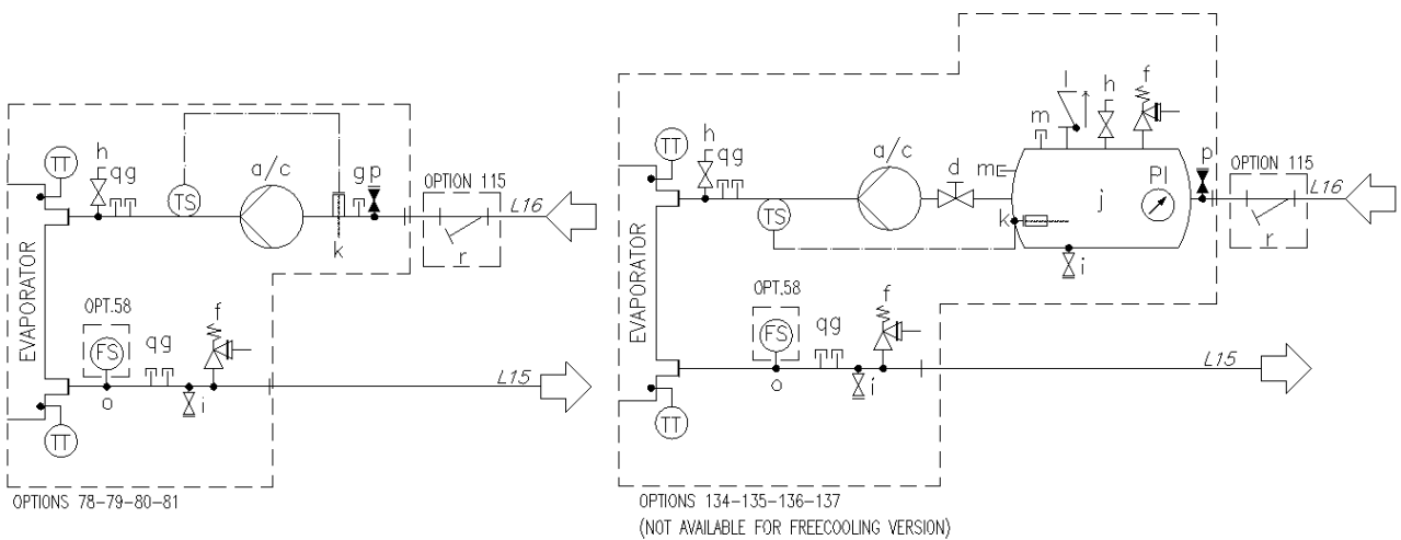
Fig. 8 - Diagrama hidráulico para Modular V (EWATxx0B) (opc. 78-79-80-81/134-135-136-137) (pressão máxima de funcionamento 6 bar)
