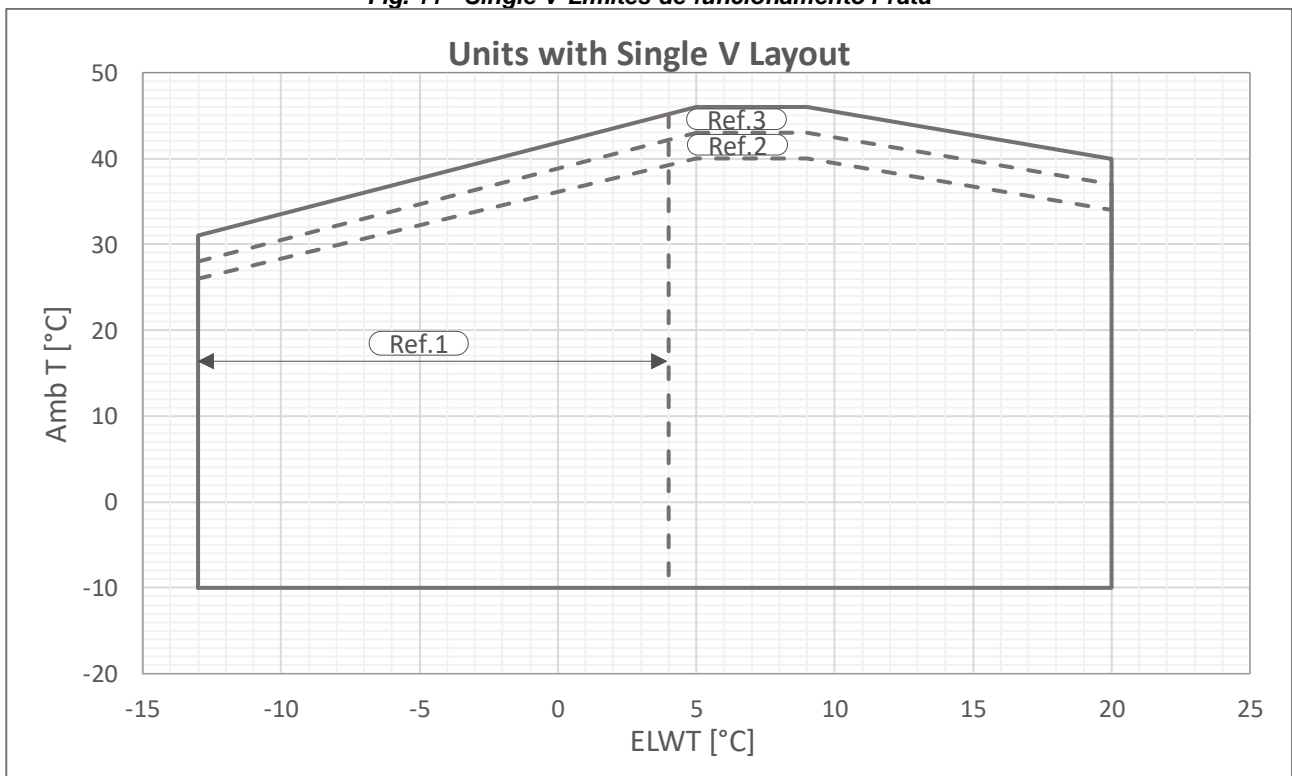
Fig. 12 - Single V-Limites de funcionamento Ouro
