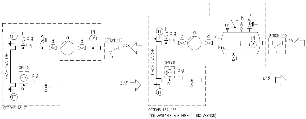
Fig. 6 - Diagrama hidráulico para bomba única V (EWATxx5B) (opc. 78-79/134-135) (pressão máxima de funcionamento 6 bar)
