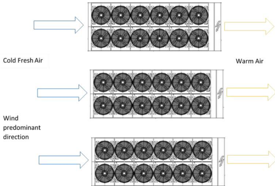
Fig. 4 - Instalação de múltiplos refrigeradores
