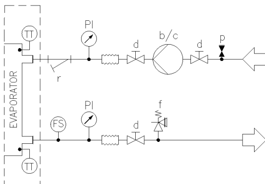
Fig. 5 - Esquema hidráulico sem bomba(s) a bordo (pressão máxima de funcionamento 20 bar)
