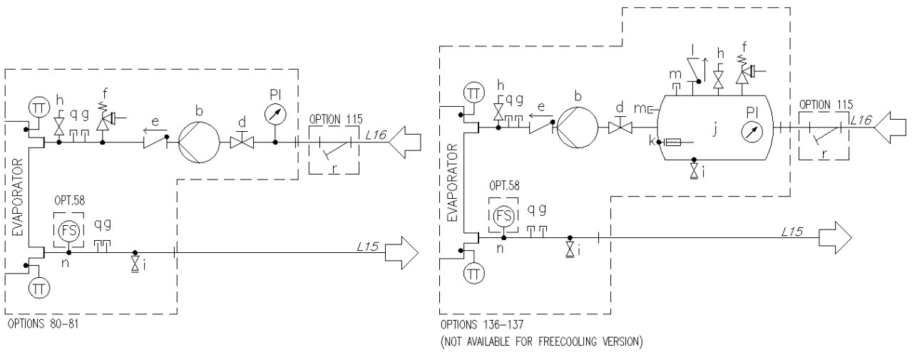
Fig. 7 - Diagrama hidráulico para bomba dupla V (EWATxx5B) (opc. 80-81/136-137) (pressão máxima de funcionamento 6 bar)
