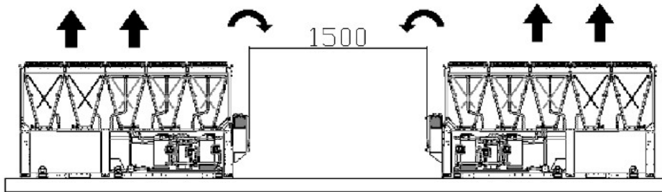
Abb. 3 - Mindestabstände
