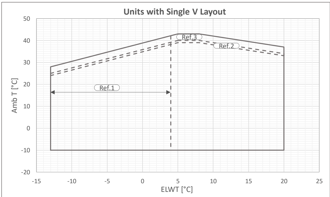
Abb. 9 - Einzelner V-Silber Betriebsgrenzen
