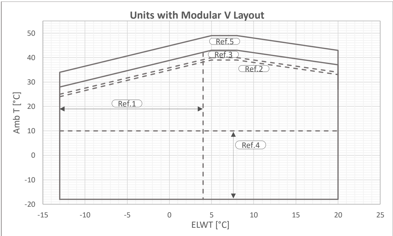
Abb. 10 - Multi-V-Silver Betriebsgrenzen
