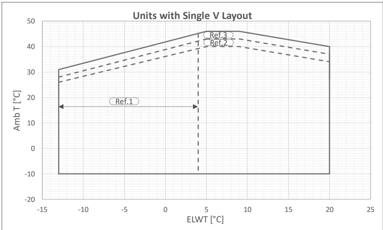
Abb. 10 - Einzelner V-Gold Betriebsgrenzen
