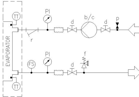
Abb. 5 – Hydraulikschema ohne eingebaute Pumpe(n) (max. Betriebsdruck 20 bar)
