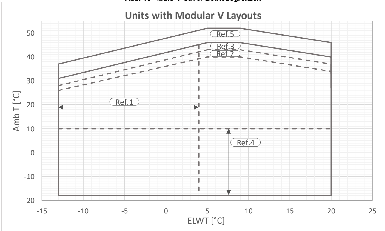
Abb. 11 - Multi-V-Gold Betriebsgrenzen
