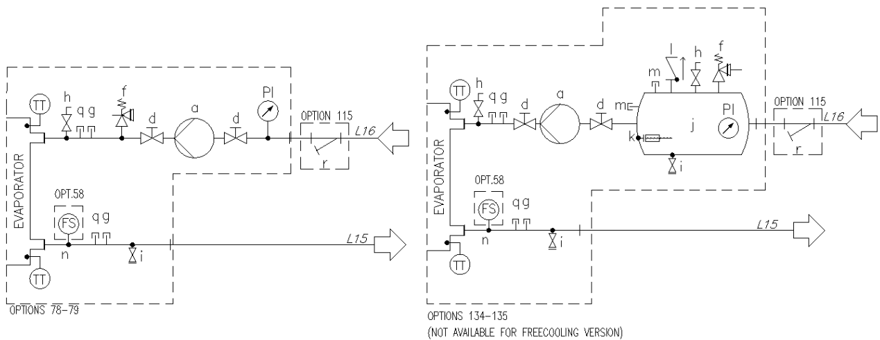
Abb. 6 – Hydraulikschema für einzelne V-Anlage (EWATxx5B) einfache Pumpe (Opt. 78-79/134-135) (max. Betriebsdruck 6 bar)
