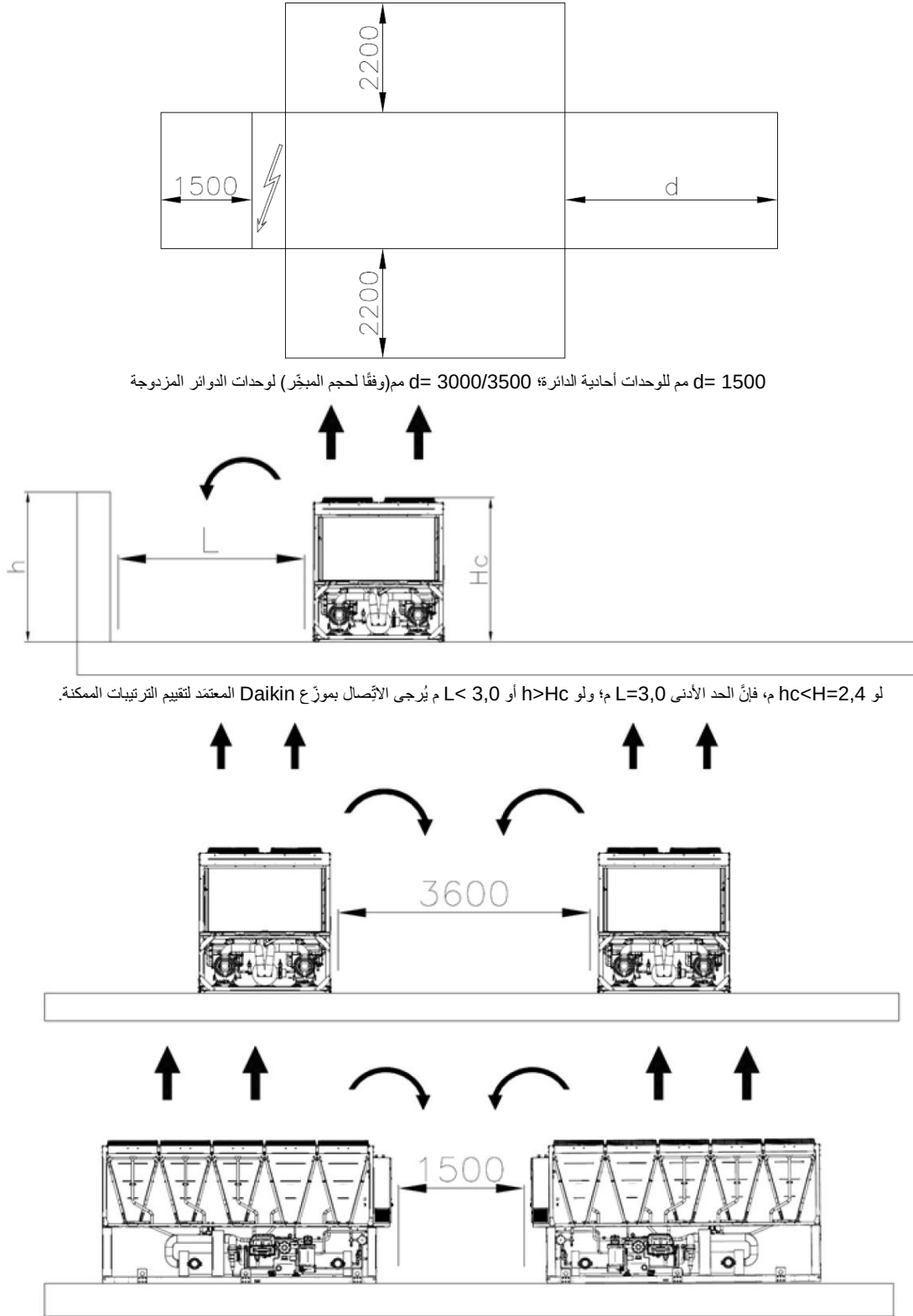
الشكل 5 - الحد الأدنى لمتطلبات الخلو
