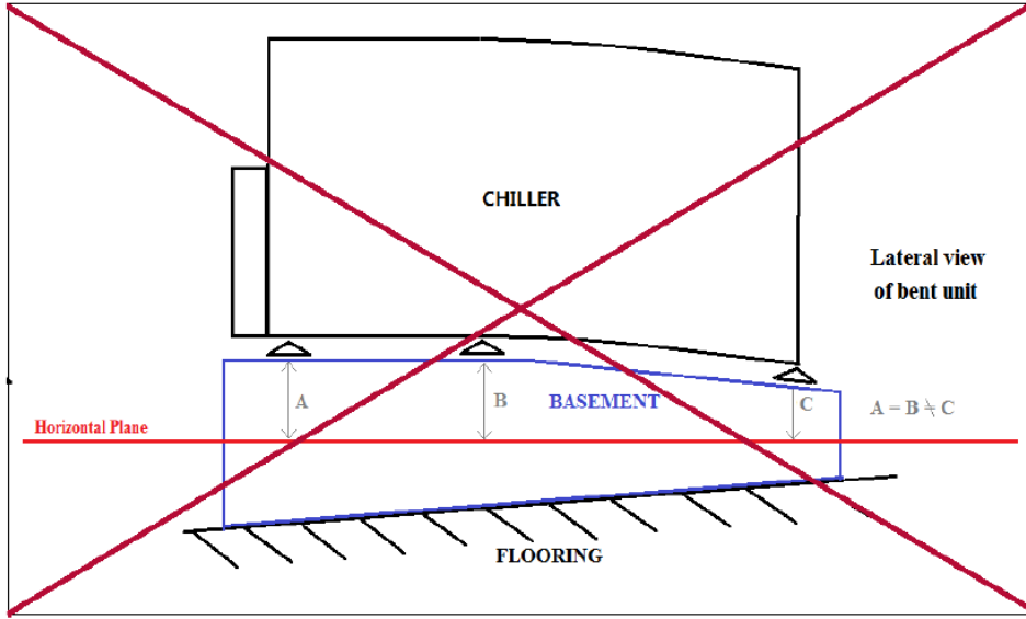
الشكل 4- ضبط استواء الوحدة
