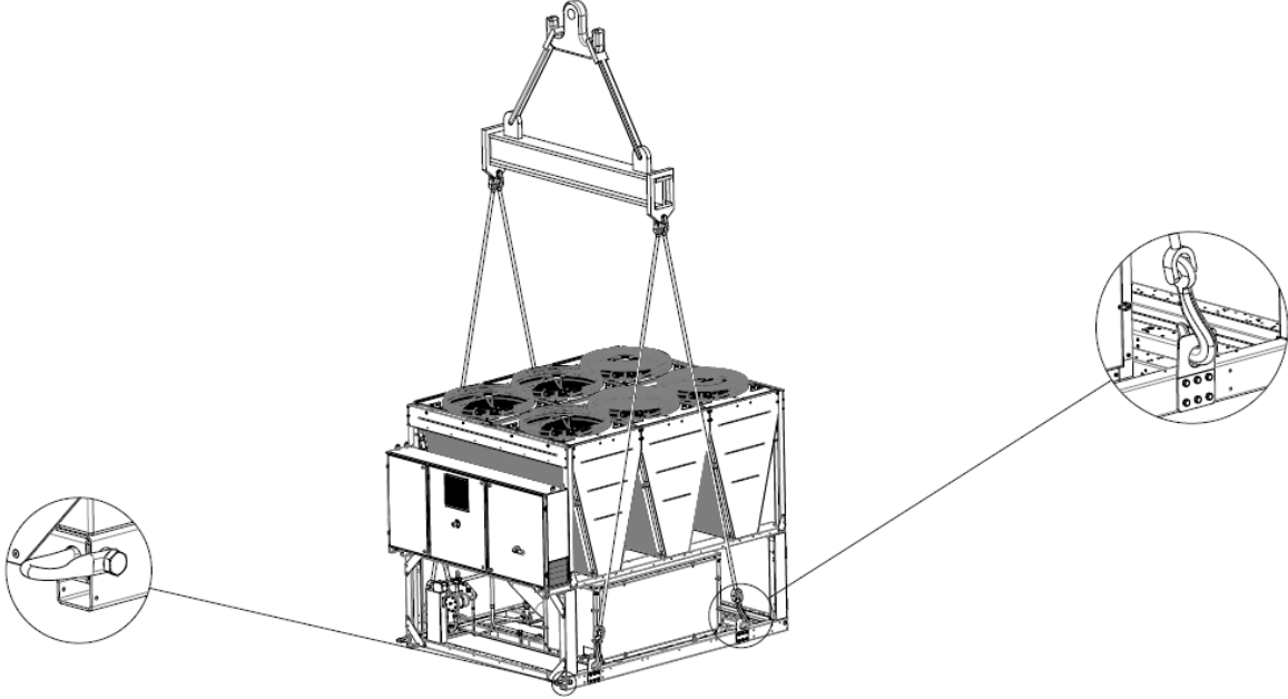
الشكل 3- رفع الوحدة وحدة بها 4 نقاط رفع
