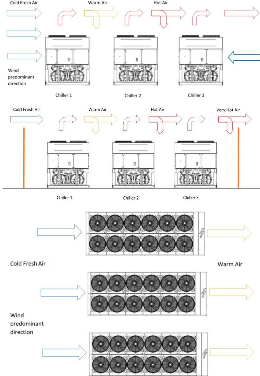
الشكل 6 – تركيب المبرد المتعدد
