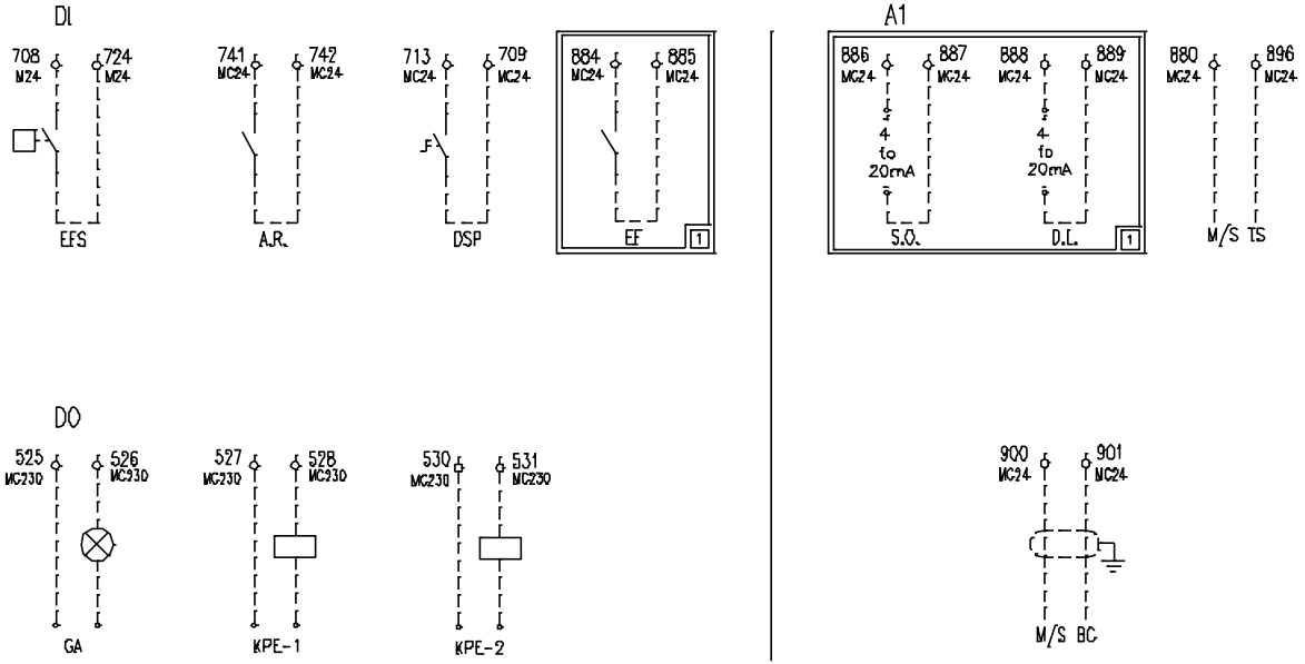
Şekil 5 – Kurulum yerindeki ünitenin kablo bağlantıları
