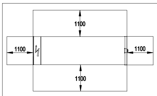
Slika 3 – Predpisane razdalje:
