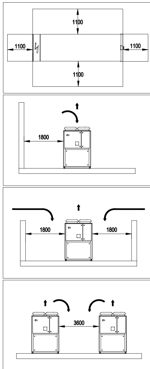
Obrázok 3 - Vzdialenosti, ktoré je potrebné dodržať
