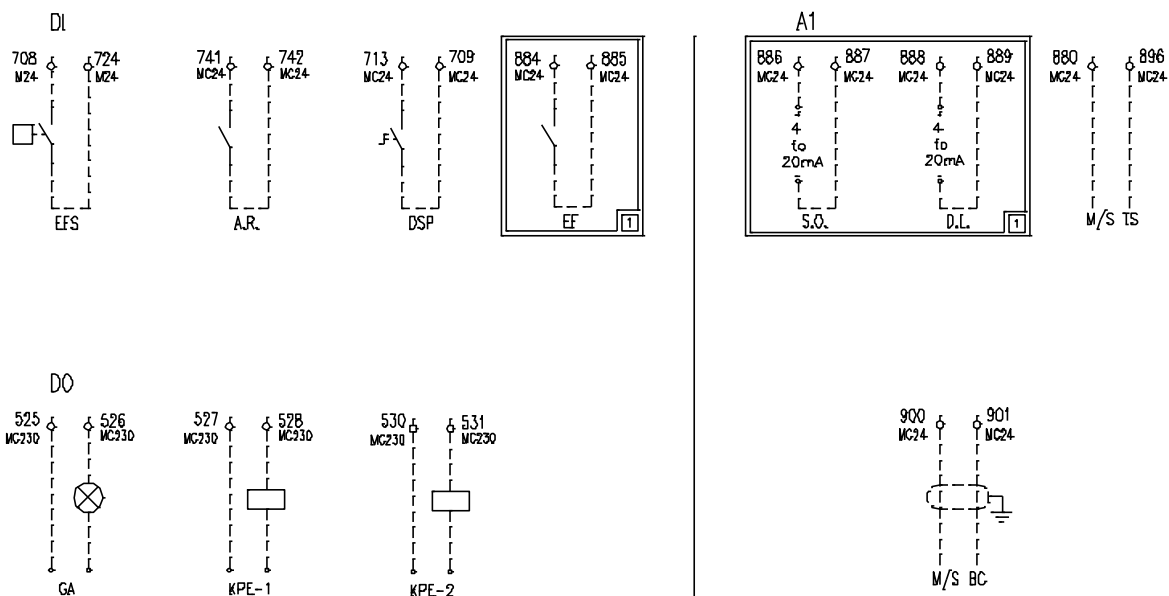
Obrázok 5 – Kabeláž jednotky na mieste inštalácie
