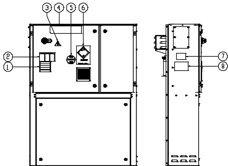
Figura 1 - Descrierea etichetelor aplicate pe panoul electric
