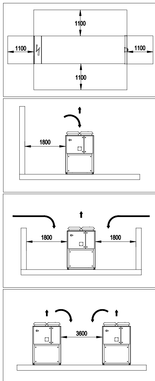
Figura 3 - Distanțe obligatorii:
