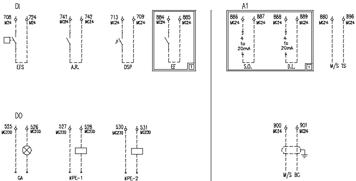
Rysunek 5 – Połączenia elektryczne jednostki w miejscu instalacji
