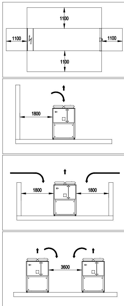
Rysunek 3 - Wymagane odległości:
