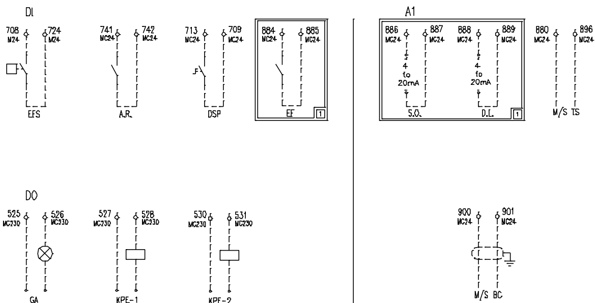
Εικόνα 5 – Καλωδίωση μονάδας στη θέση εγκατάστασης
