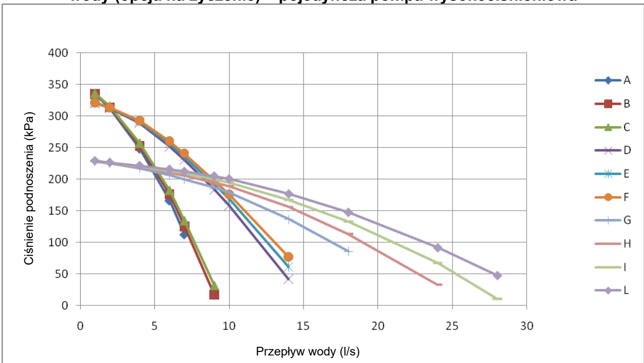
Rysunek 12 – EWAD E-SS/SL – dostępny zestaw zewnętrznego ciśnienia dla pomp wody (opcja na życzenie) – pojedyncza pompa wysokociśnieniowa
