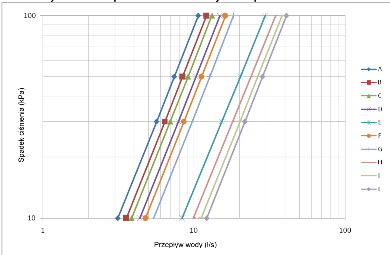
Rysunek 16 – spadek ciśnienia w odzysku ciepła – EWAD E-SS/SL
