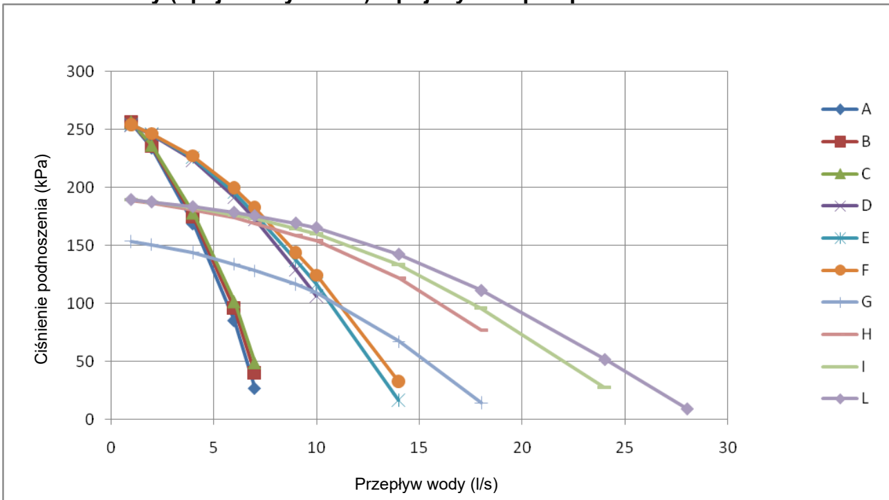
Rysunek 11 – EWAD E SS/SL – dostępny zestaw zewnętrznego ciśnienia dla pomp wody (opcja na życzenie) – pojedyncza pompa niskociśnieniowa
