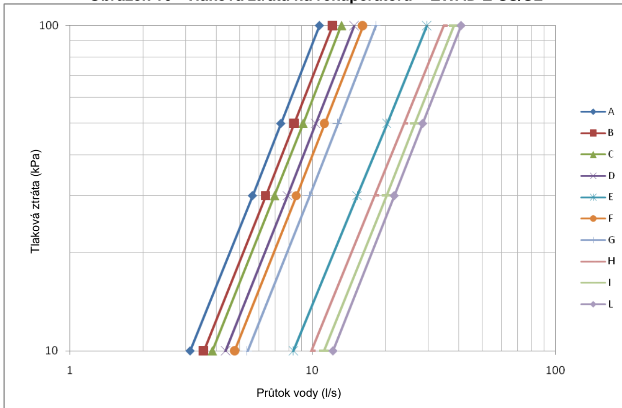
Obrázek 16 - Tlaková ztráta na rekuperátoru – EWAD E-SS/SL
