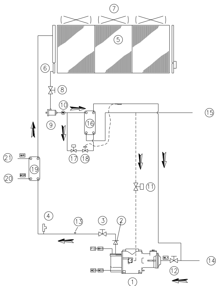
Obrázek 25 – ERAD120E ÷ 490E-SS – ERAD 120E ÷ 460E-SL Okruh chladiva s rekuperací tepla – jednotky bez ekonomizéru
