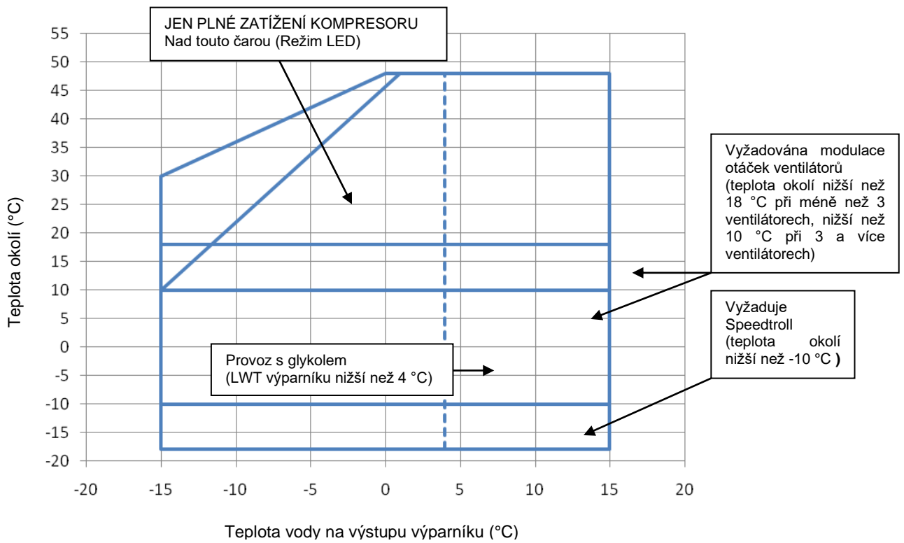
Obrázek 3 - Provozní limity – ERAD E-SS/SL
