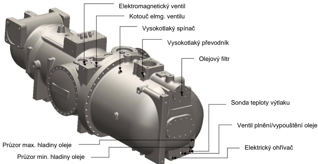
Obrázek 33 - Instalace řídicích prvků kompresoru F3
