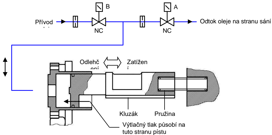
Obrázek 30 - mechanismus řízení kapacity kompresoru Fr3100
