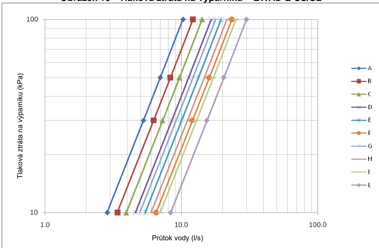
Obrázek 15 - Tlaková ztráta na výparníku – EWAD E-SS/SL
