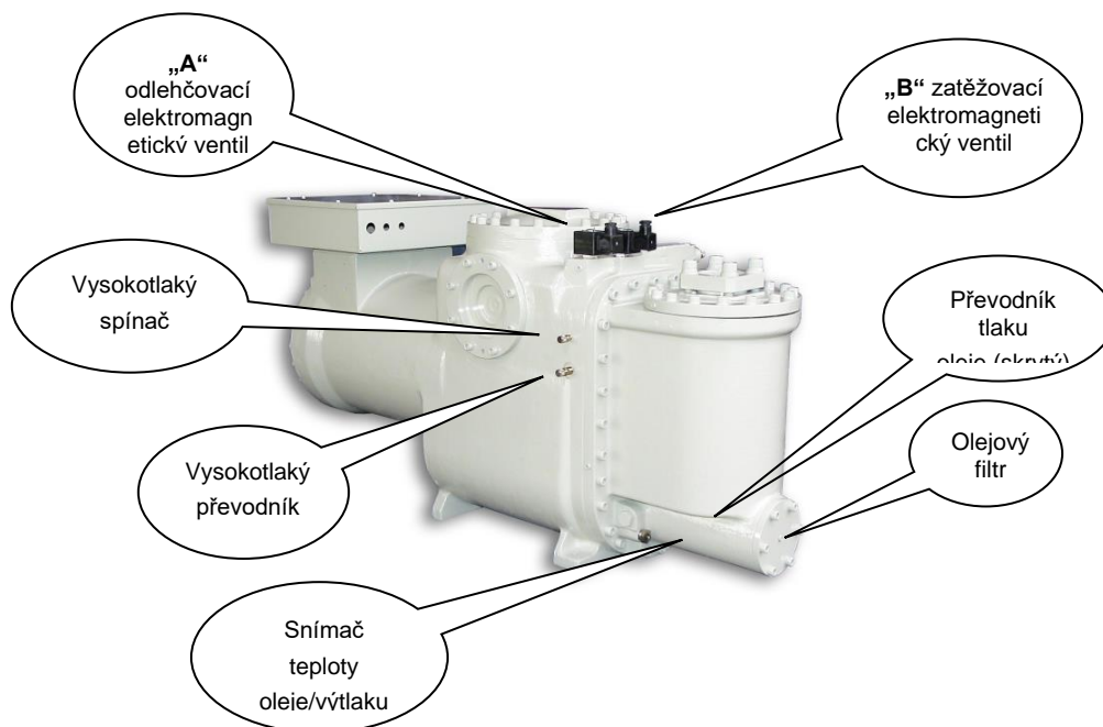
Obrázek 32 - Instalace řídicích prvků kompresoru Fr3100
