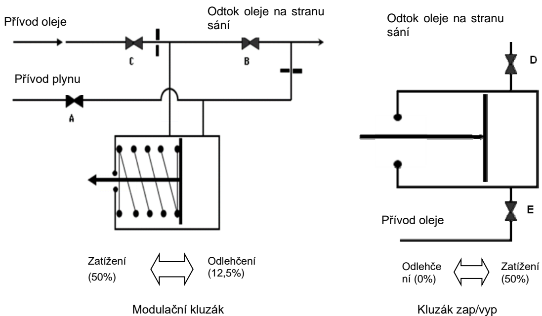
Obrázek 31 - mechanismus řízení kapacity kompresoru F3
