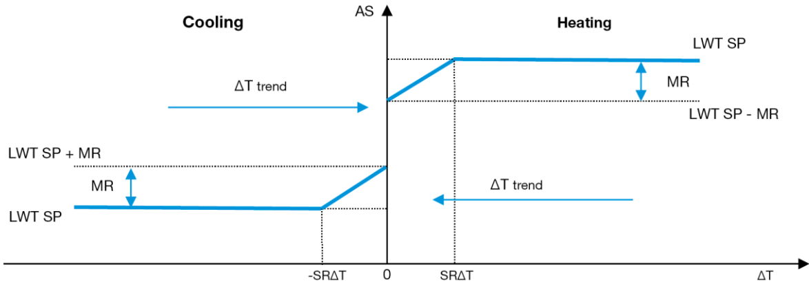
Grafiek 5 – Verdampers \Delta T tegen Actief Setpoint - Modus Koelen (links) / Modus Verwarmen (rechts)
