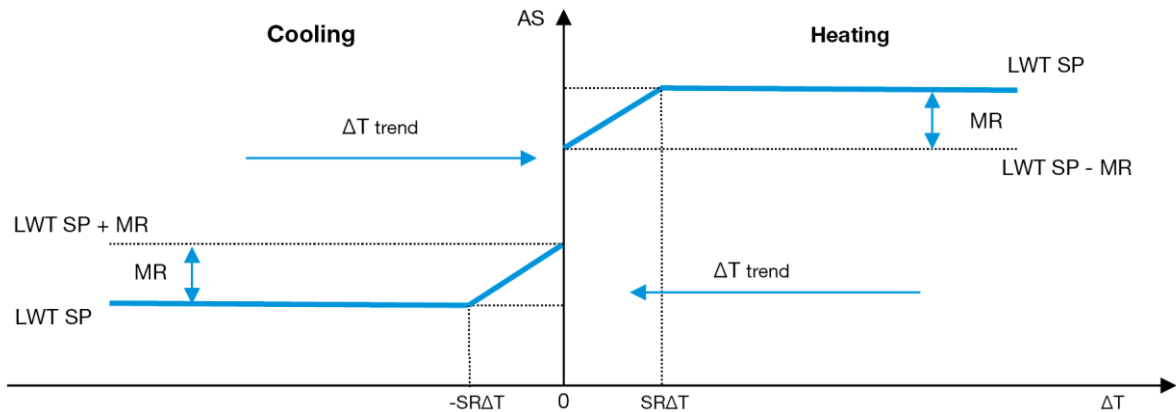
5. grafikon – Párol. \Delta T vs Aktív beállítási pont - Hűtés mód (balra)/Fűtés mód (jobbra)
