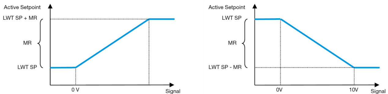
Gráfico 4– Señal externa de 0-10V contra Punto de Ajuste Activo - Modo de enfriamiento (izquierda)/ Modo de calentamiento (derecha)
