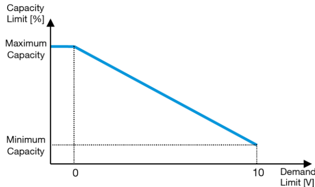
Diagramm 2 – Bedarfsbegrenzung [mA] gegenüber Kapazitätsgrenze [%]
