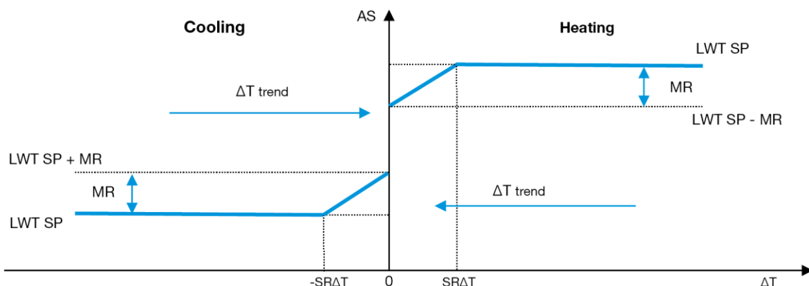
Graphique 3 –Evap \Delta T vs. Point de consigne actif - Mode de refroidissement (à gauche) / Mode de chauffage (à droite)
