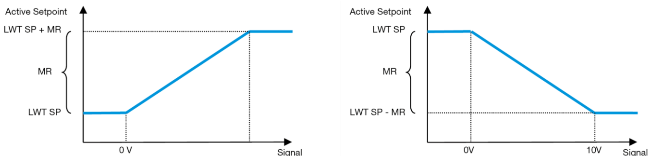
Wykres 4 – Sygnał zewnętrzny 0-10V a Aktywna nastawa - w trybie chłodzenia (wykres lewy) lub ogrzewania (wykres prawy)
