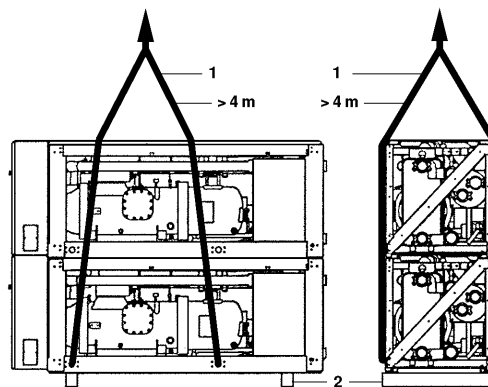
Figura 3– Elevación
