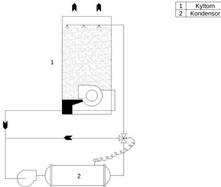
Figur 11 - Kondensorns kontrollschemat med kyltorn
