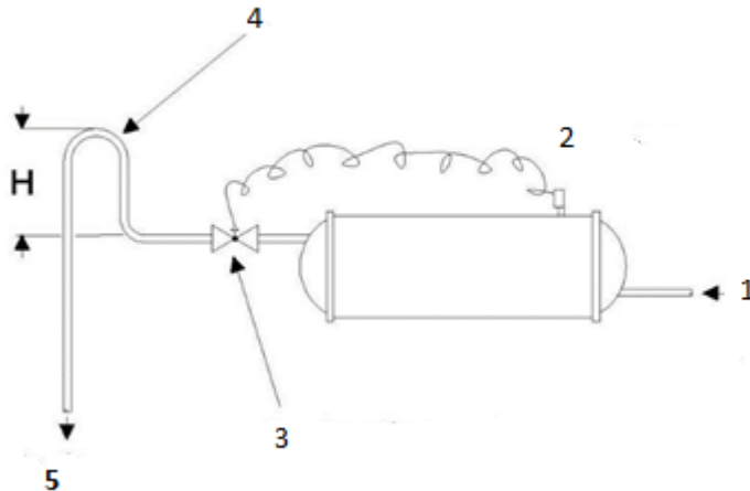
Figur 12 - Kondensorns kontrollschema med behållarvatten
