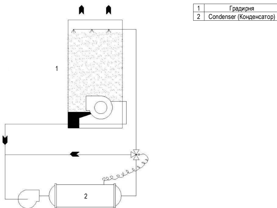
Рис. 11. Схема управления конденсатором с градирней
