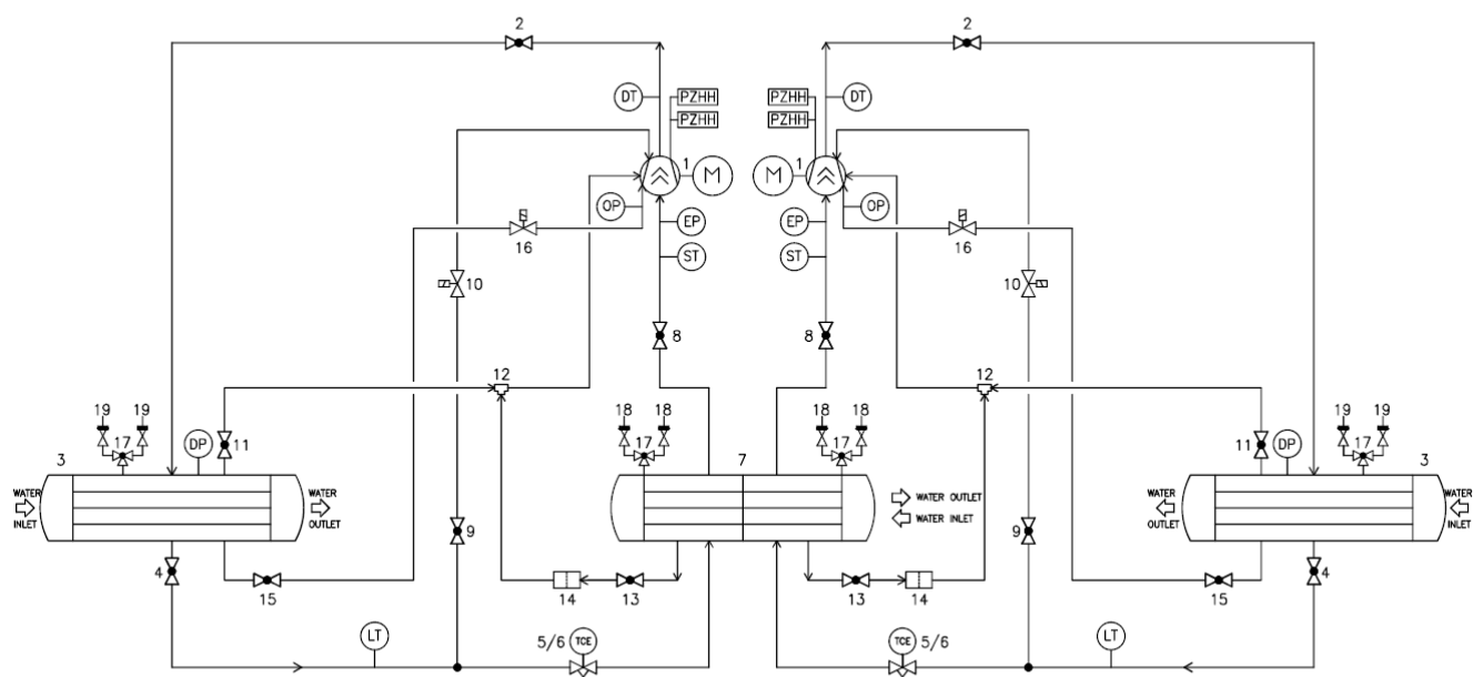
Рис. 15. Типовой двухконтурный контур охлаждения
