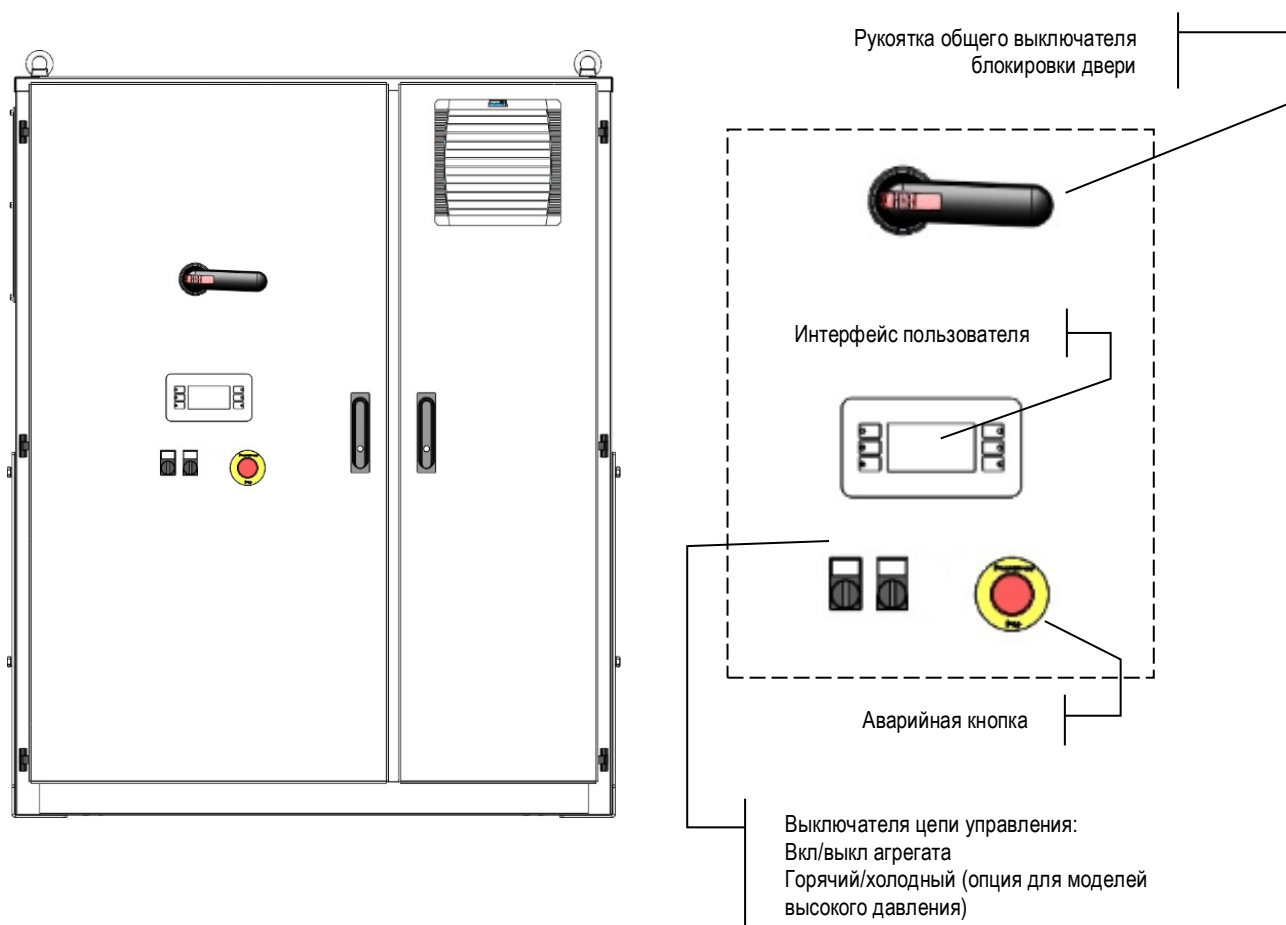
Рис. 13. Интерфейс агрегата
