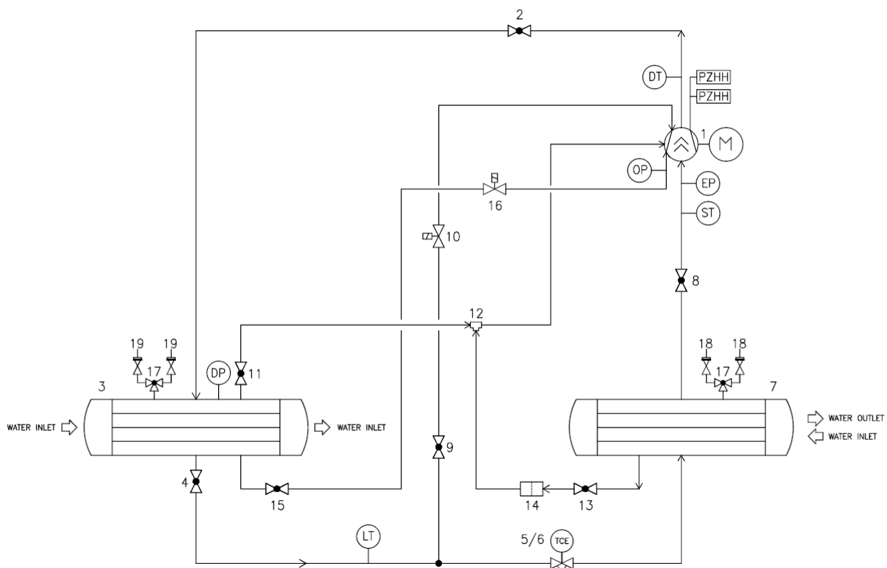
Рис. 14. Типовой одноконтурный контур охлаждения
