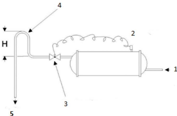
Рис. 12. Схема управления конденсацией при использовании артезианской воды
