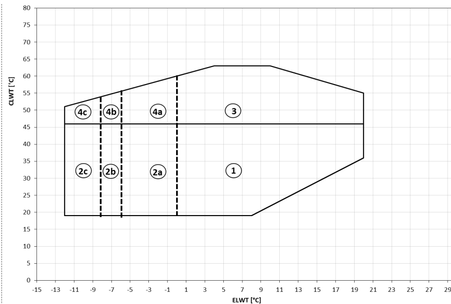
Рис. 5. Рабочий диапазон EWWD_VZ_SS
