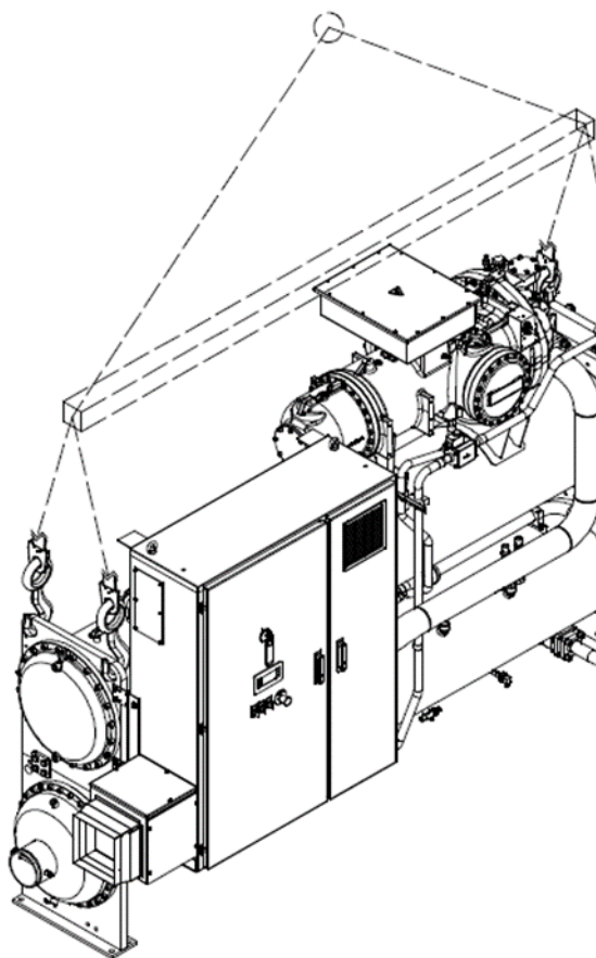
Одноконтурный агрегат
