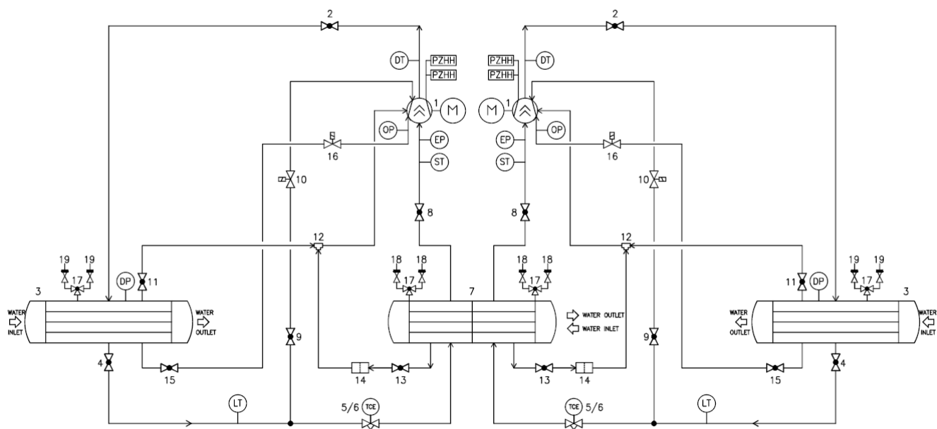
Rys. 15 - Typowy obieg chłodzenia podwójnego obiegu
