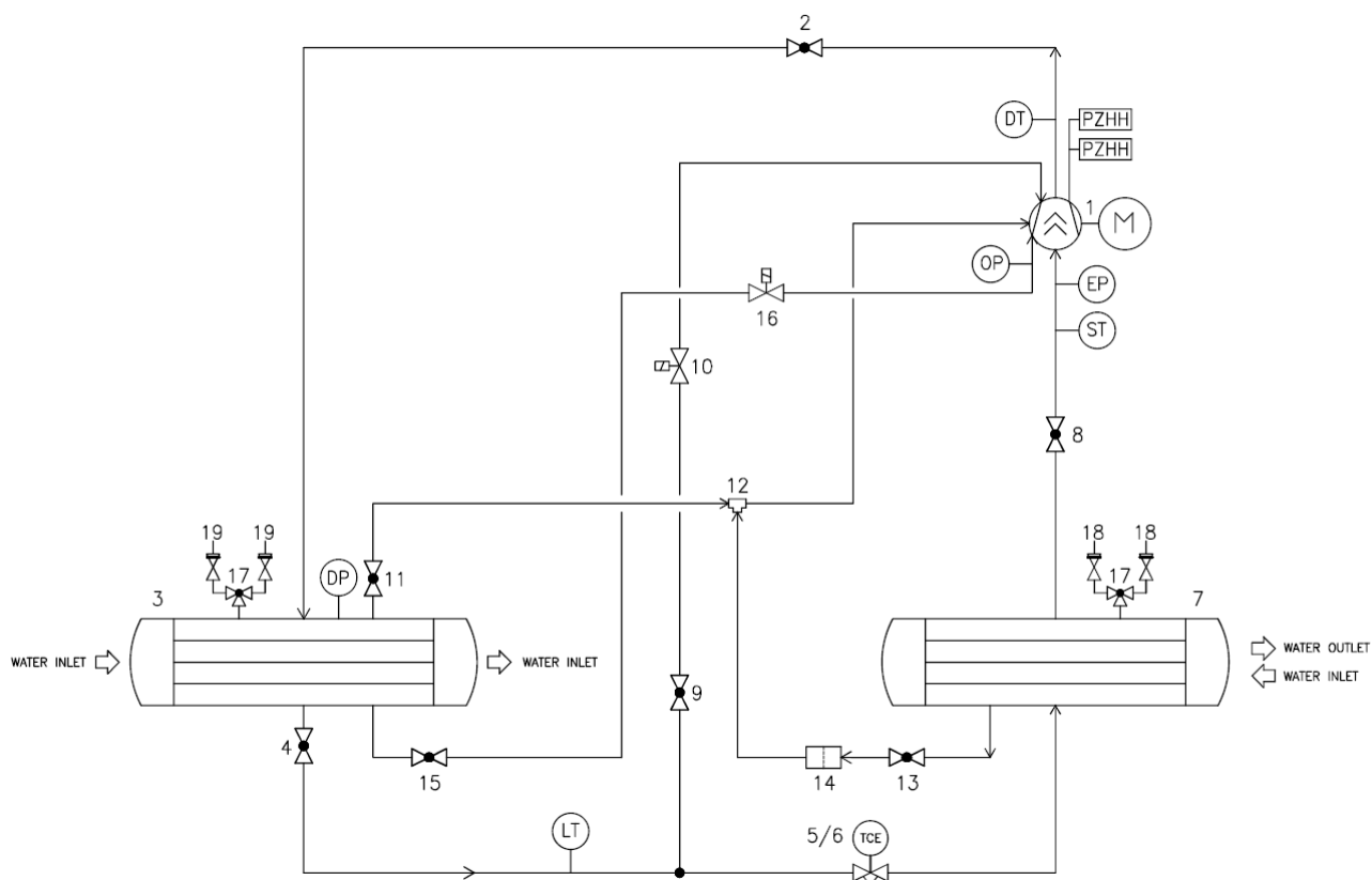
Rys. 14 - Typowy obieg chłodzenia pojedynczego obiegu
