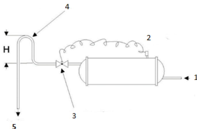
Rysunek 12 - Schemat kontroli skraplacza za pomocą wody źródlanej
