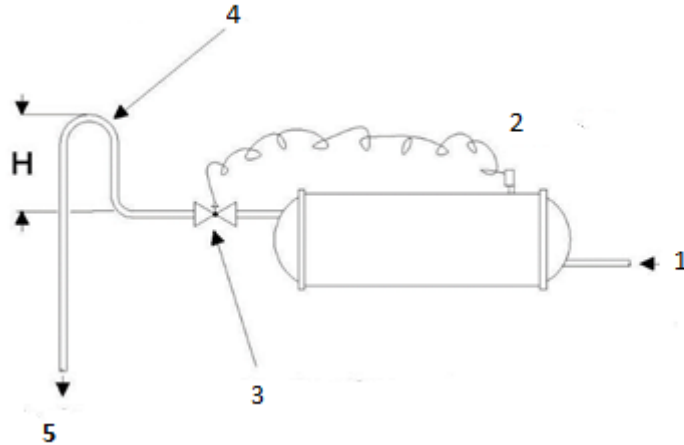
Afbeelding 12 -Regelschema condensatie met bronwater
