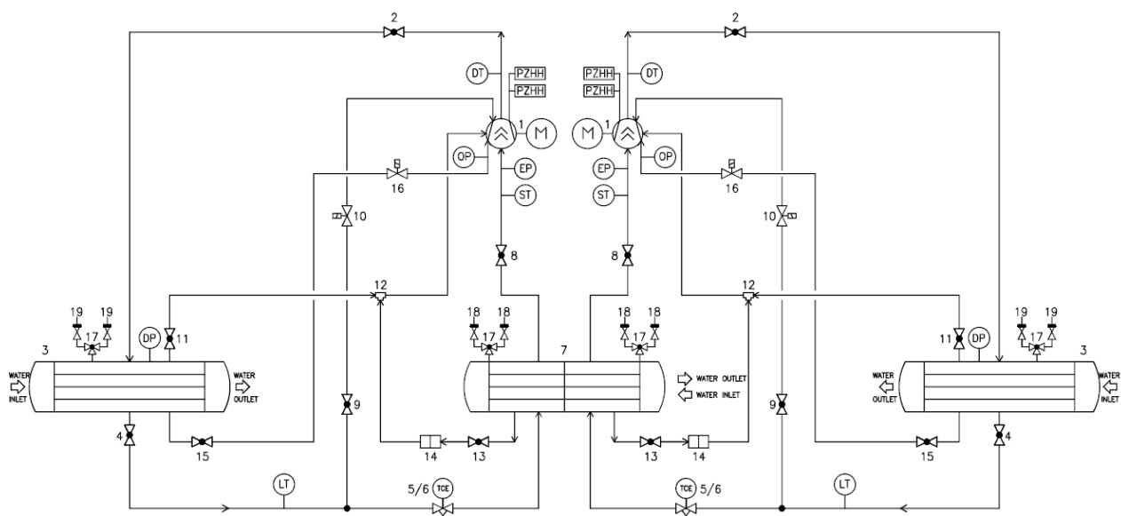
Afbeelding 15 - Typisch koelcircuit met dubbel circuit
