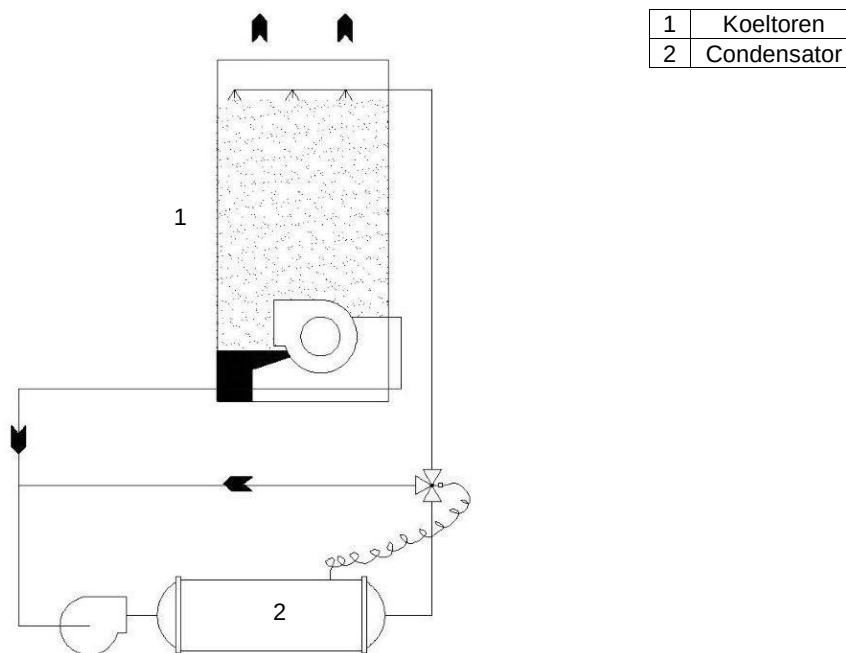
Afbeelding 11 – Regelschema condensator met koeltoren
