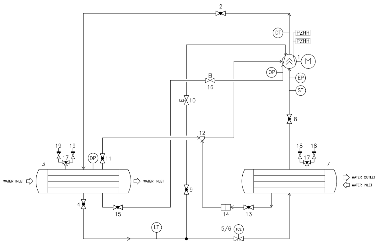
Afbeelding 14 - Typisch koelcircuit met één circuit
