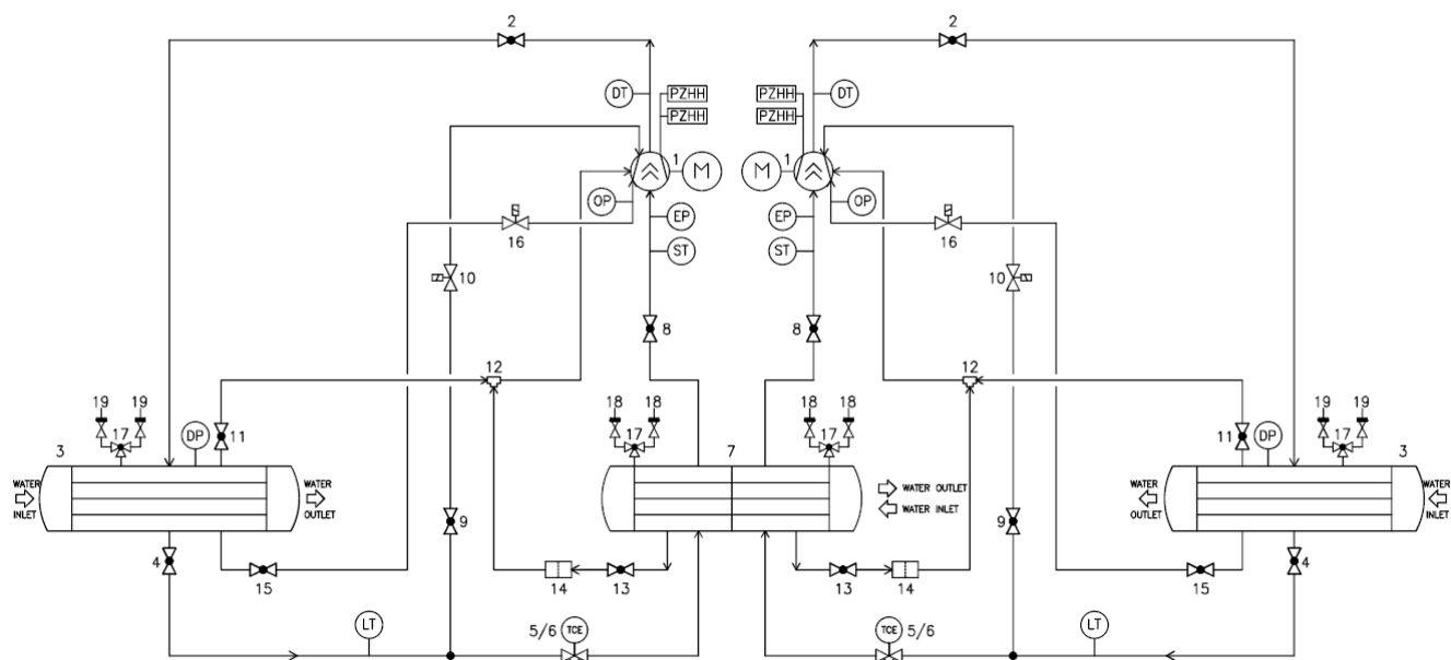
Obrázek 15 – Typický okruh chlazení se dvěma okruhy
