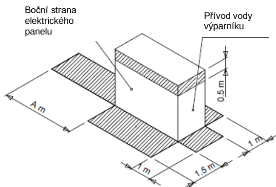
Obrázek 4 – Vybavení jednotky
