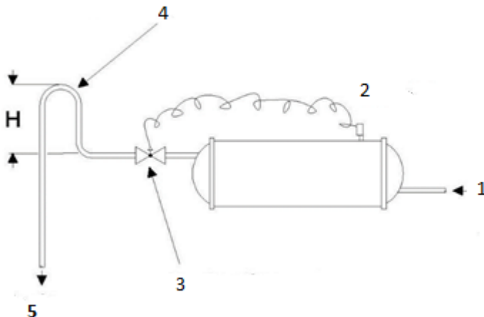
Obrázek 12 – Systém řízení kondenzace podpovrchovou vodou
