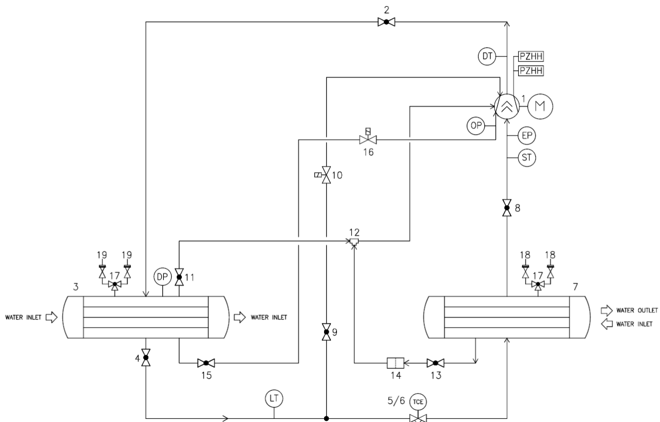
Obrázek 14 – Typický okruh chlazení jednoho okruhu
