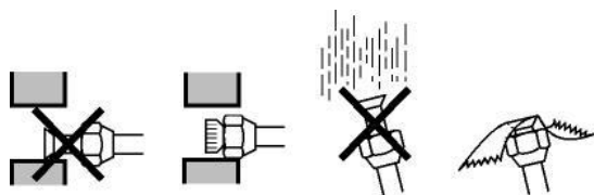
Figura 6- Connessione del circuito refrigerante (4)
