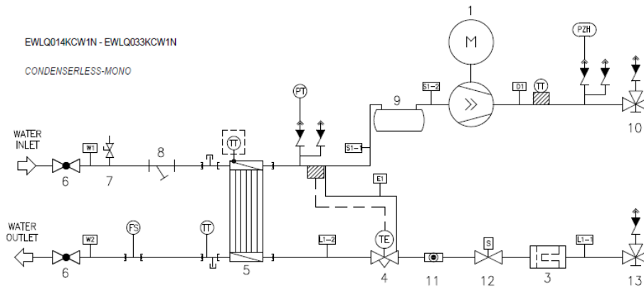
Figura 12- EWLQ 049 - 064 KCW1N Schema circuito refrigerante
