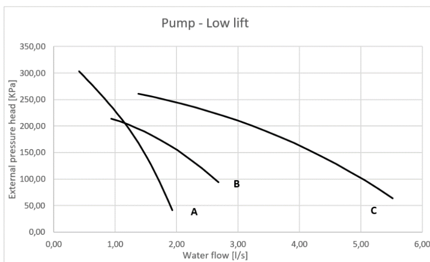
Figura 16 – Cabeça de pressão externa da bomba de água
