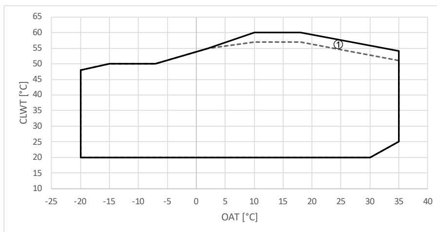
Figura 18 – Limites de operação no EWYTCZ no modo de aquecimento
