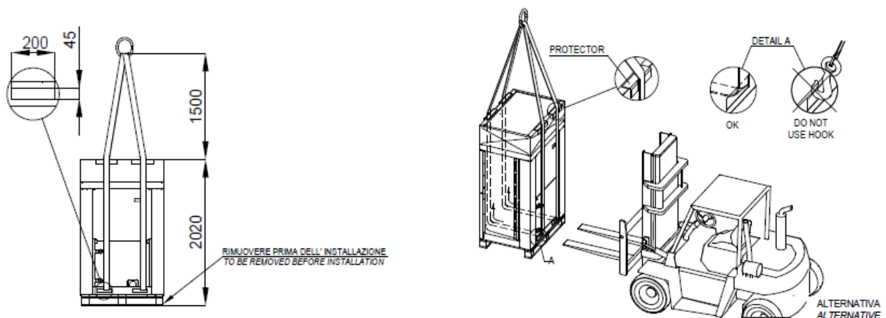
Figura 1 – Elevação da unidade MONO externa
