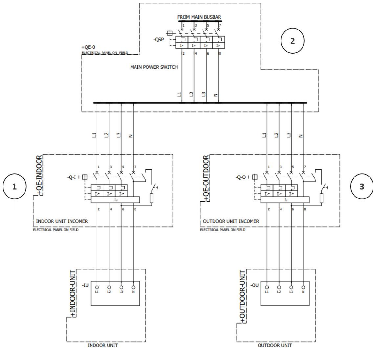
Figura 21 – Diagrama de ligações principal
