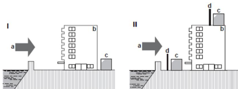
Figura 11 – Instalação à beira-mar da unidade exterior
