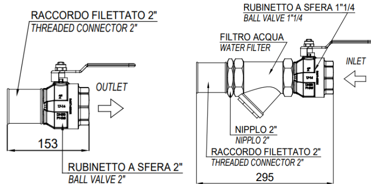
Figura 14 – Elementos hidráulicos
