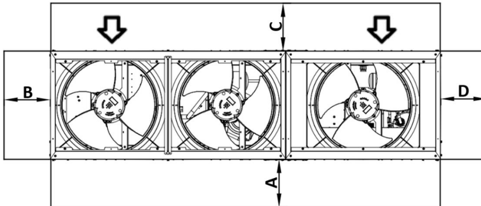
Figura 7 – Unidade DUAL
