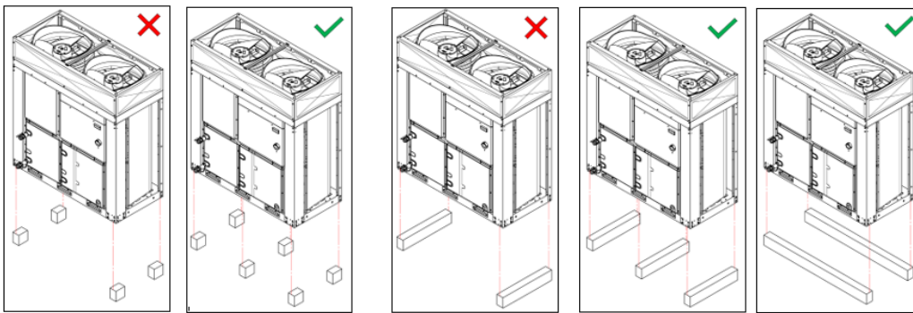
Figura 4 – Posicionamento da unidade MONO
