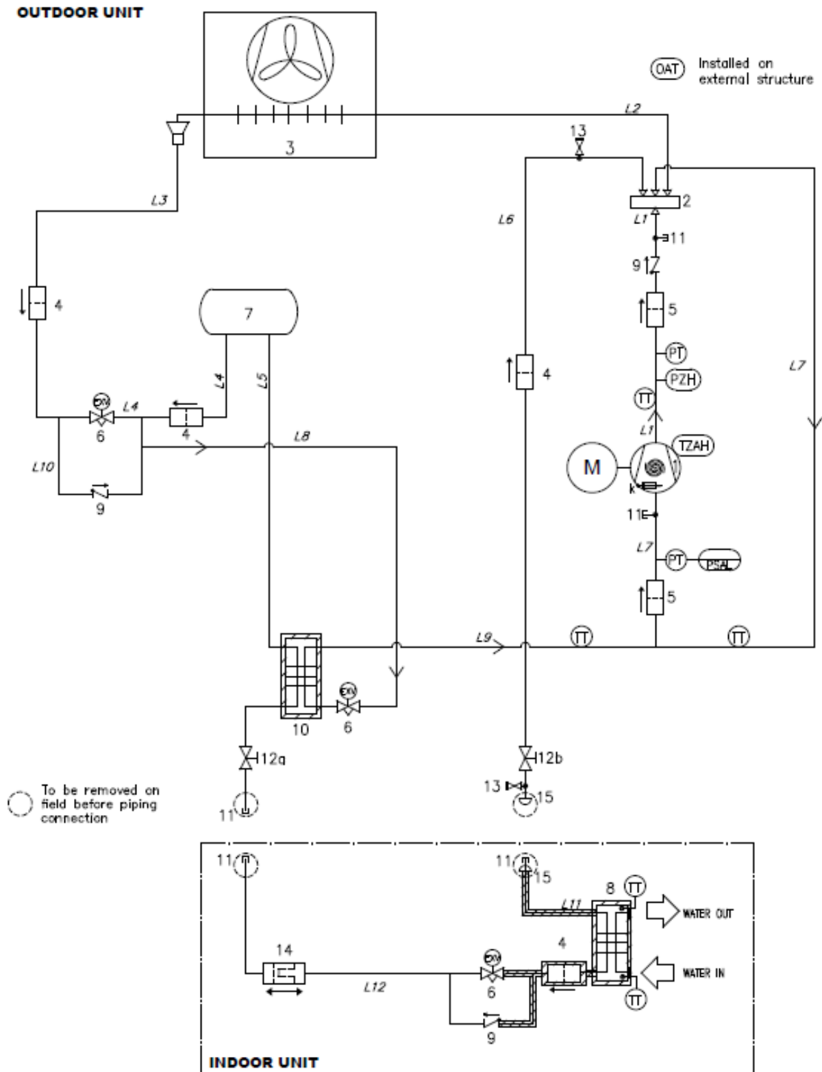
Figura 24 – Esquema do circuito de refrigeração (P&ID) para a unidade EWYT-CZ circuito MONO
