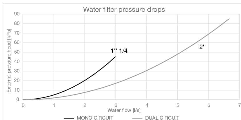
Figura 15 - Queda de pressão no filtro de água
