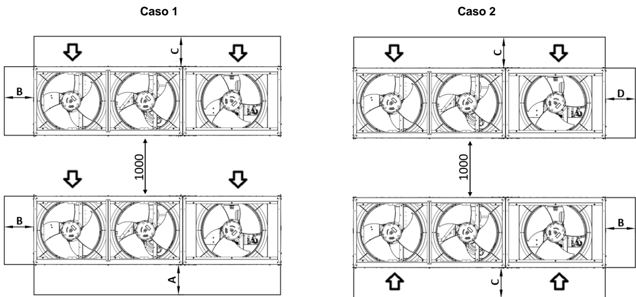
Figure 9 – Unidades instaladas lado-a-lado ao longo dos lados mais longos (Caso 1 e Caso 2)
