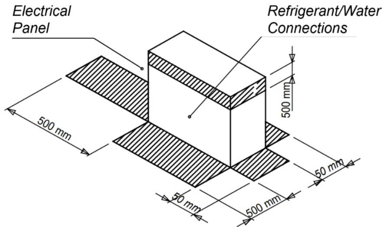
Figura 10 – Requisitos de espaço mínimo da Unidade Interior
