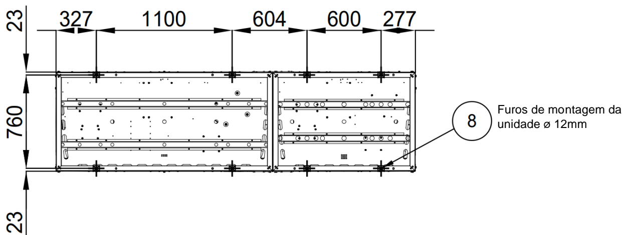
Figura 6 – Localização dos orifícios de montagem (vista inferior)
