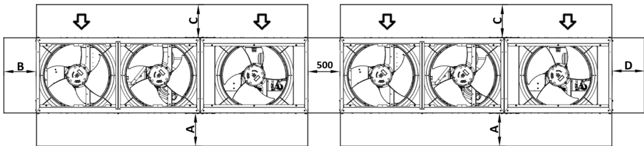
Figura 8 – Unidades instaladas lado-a-lado ao longo dos lados mais curtos, B ou D
