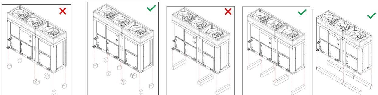
Figura 4 – Posicionamento da unidade MONO
