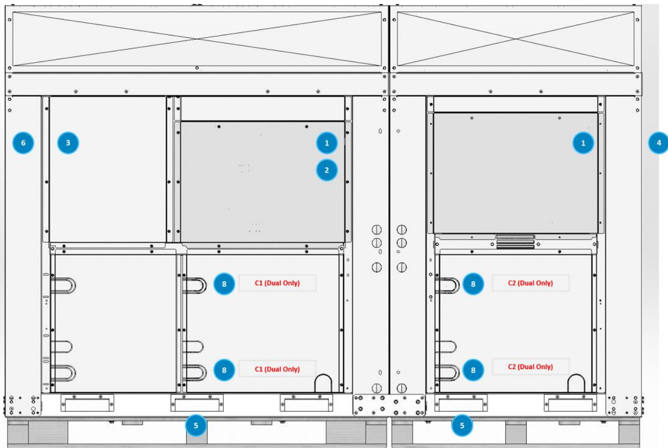
Figura 28 – Etiquetas na unidade exterior
