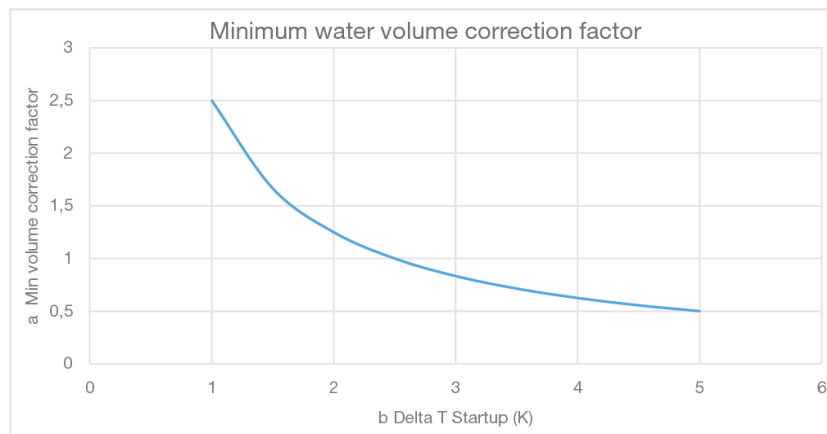
Figura 19 – Fator mínimo de correção do volume de água
