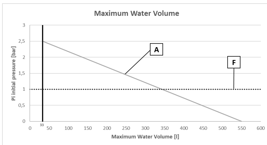
Figura 20 – Pressão inicial do vaso de expansão com base no volume máximo de água
