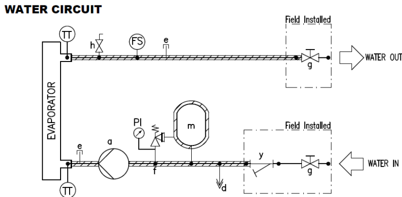
Figura 13 – Esquema hidráulico
