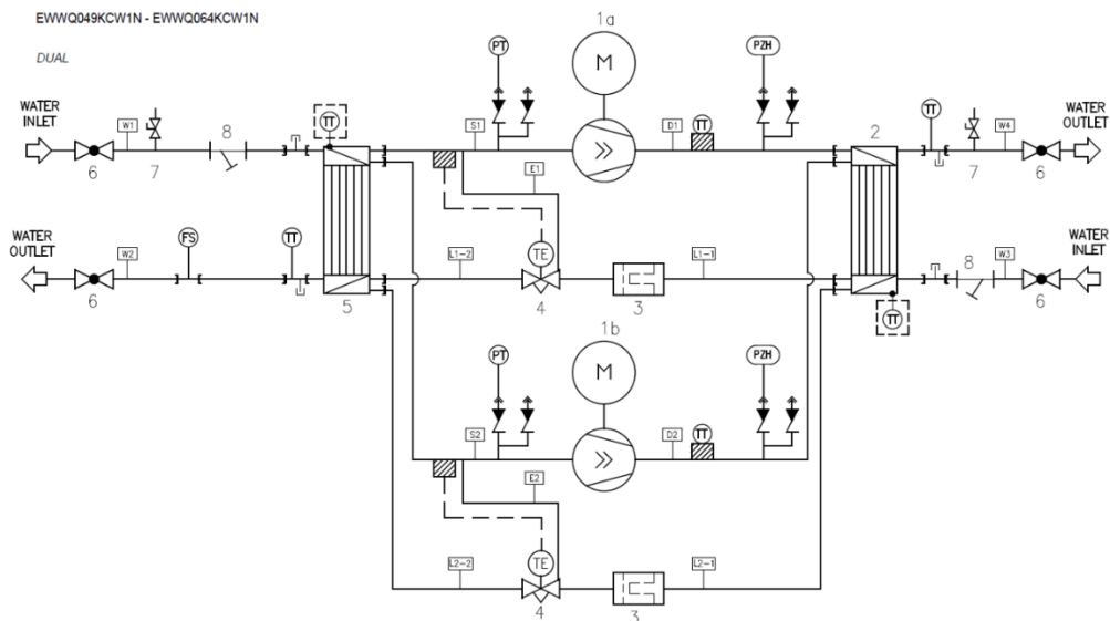
Figura 4 - Esquema do circuito de refrigerante EWWQ 049 - 064 KCW1N
