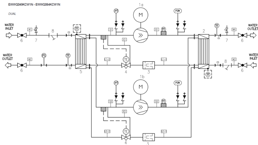
Abbildung 4 - Kältemittelkreislauf-Schema EWWQ 049 - 064 KCW1N
