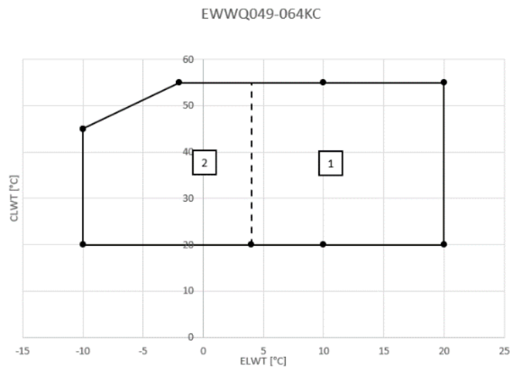
Abbildung 2 - Betriebsgrenzen EWWQ049-064
