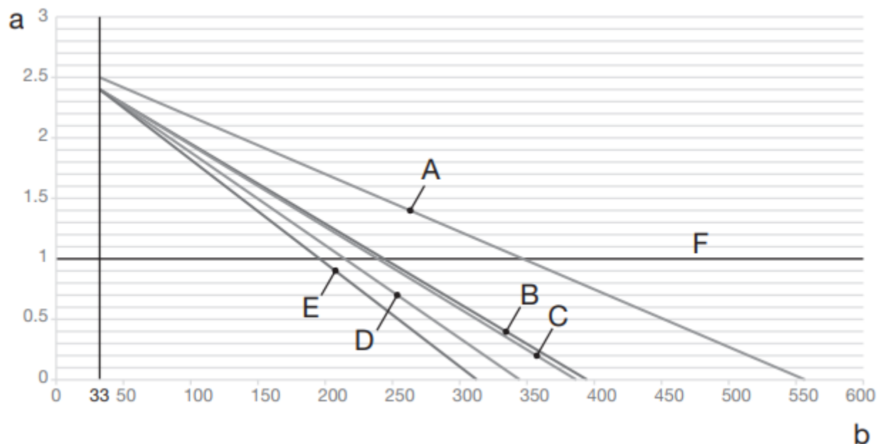
Рис. 18 - Начальное давление в расширительном баке на основе максимального объема воды
