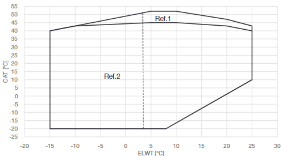
Рис. 14 – Эксплуатационные пределы на EWATCZ
