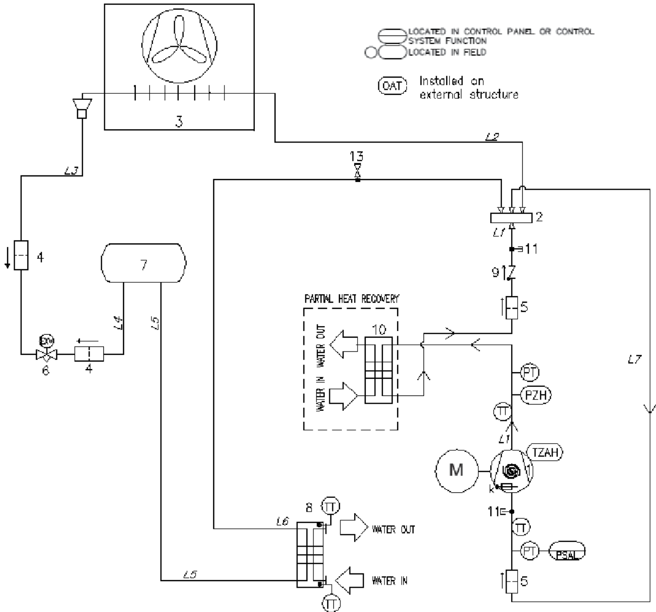
Рис. 19 - Схема контура хладагента (СТИКИП) для контура агрегата с одним контуром EWYT-CZ
