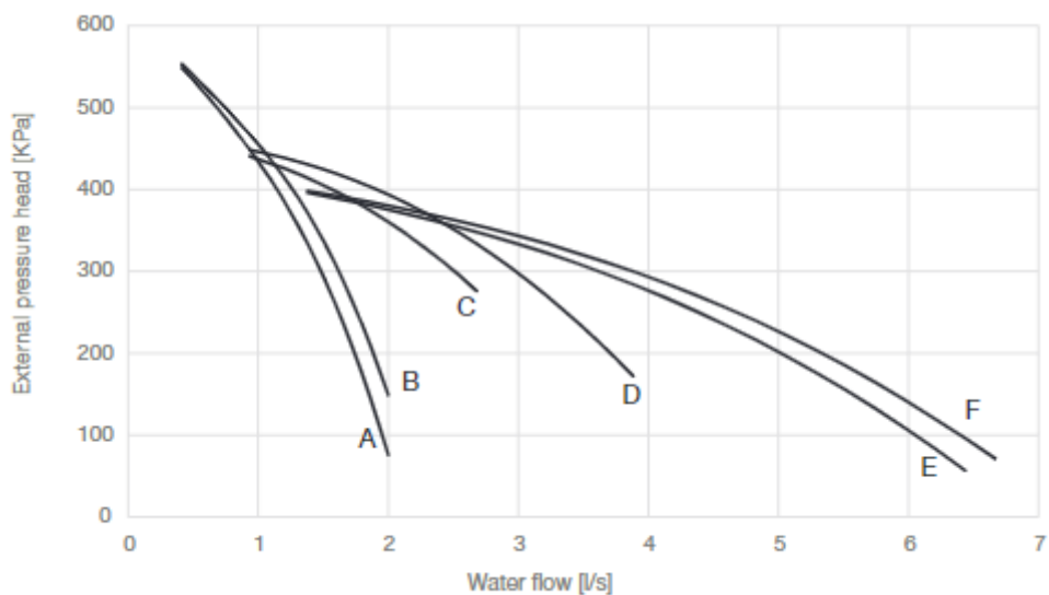
Рис. 13 - Внешний напор насоса высокого подъема
