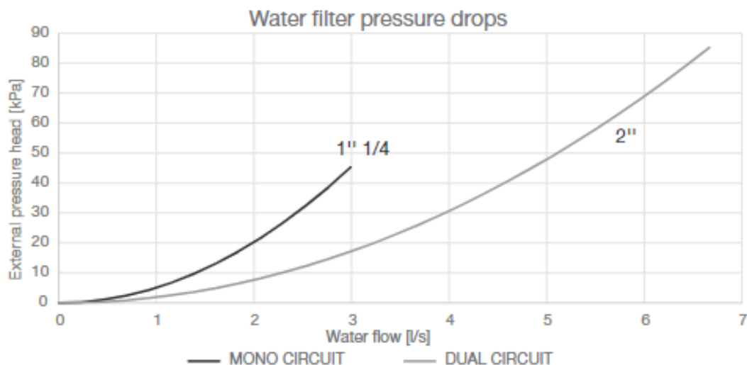
Рис. 11 - Перепад давления на фильтре для воды
