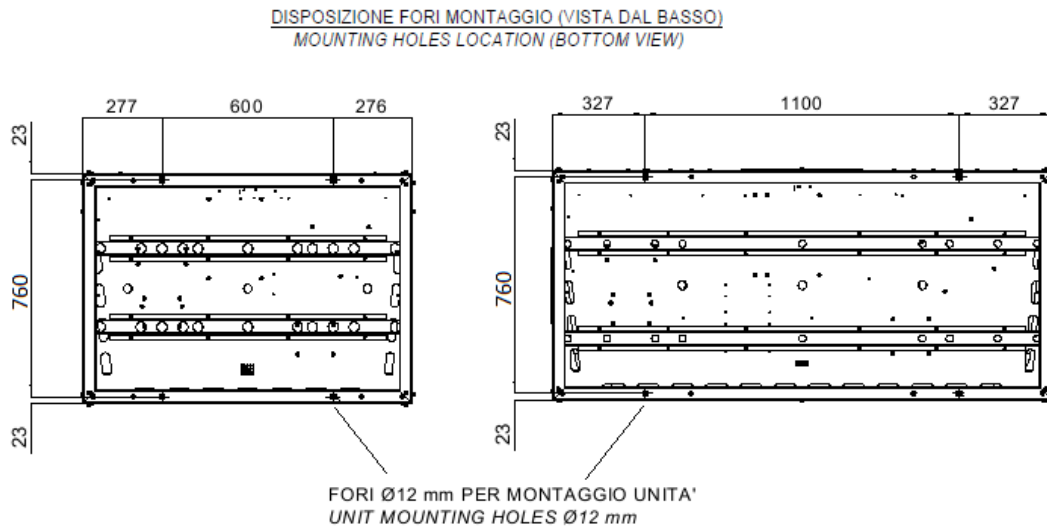
Рис. 5 – Расположение монтажных отверстий (вид снизу)
