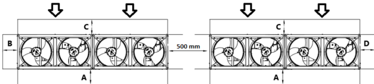
Рис. 7 –Агрегаты, установленные рядом друг с другом вдоль коротких сторон, B или D
