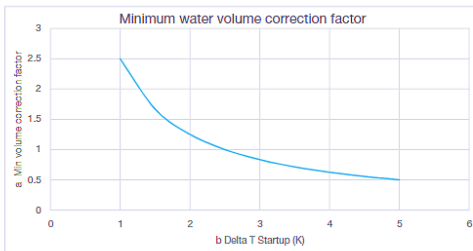
Рис. 17 - Минимальный поправочный коэффициент объема воды
