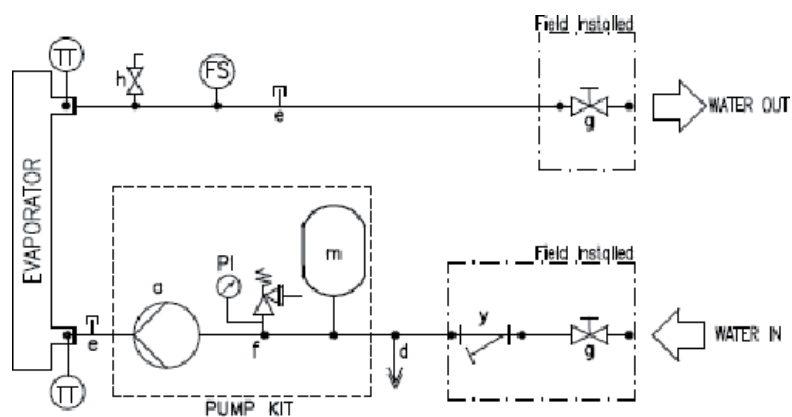
Рис. 10 –Гидравлическая схема
