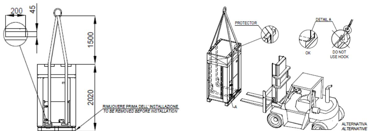
Рис. 1 – Подъем агрегата с одним контуром
