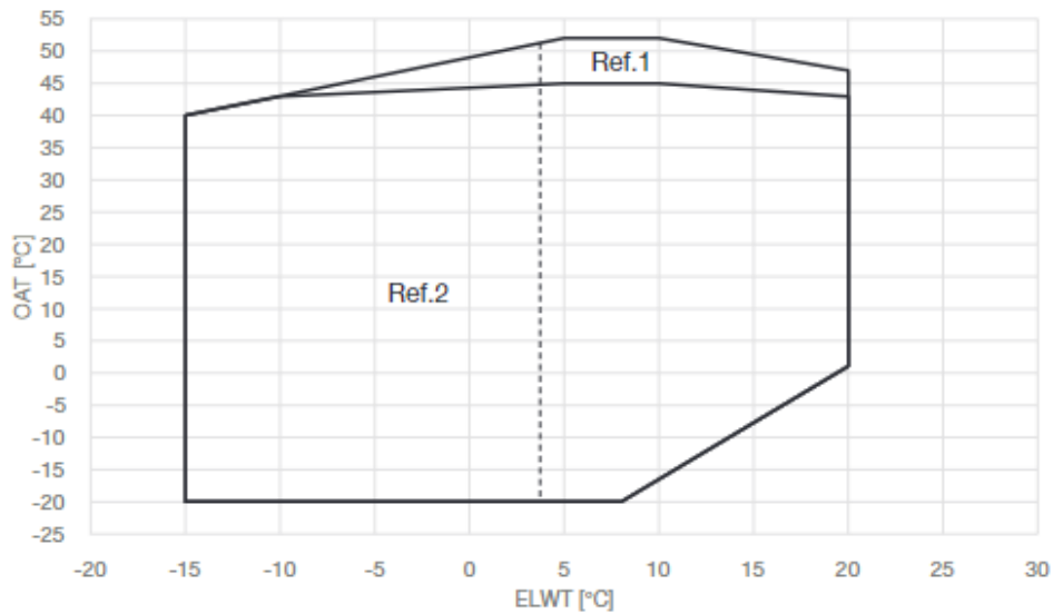
Рис. 15 - Эксплуатационные пределы для EWYTCZ в режиме охлаждения
