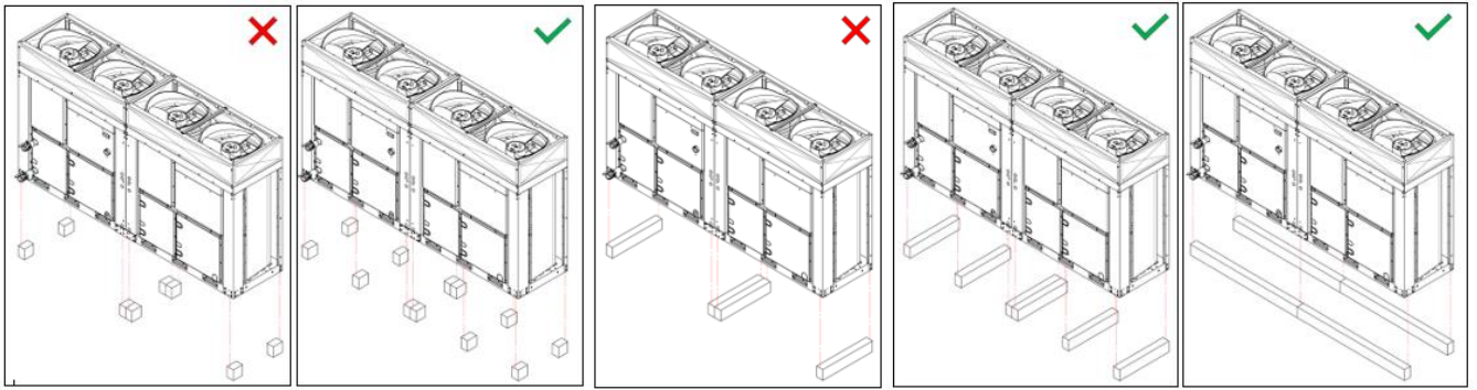
Рис. 4 – Расположение агрегата с двумя контурами
