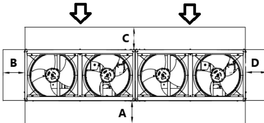
Рис. 6 – Агрегат с двумя контурами
