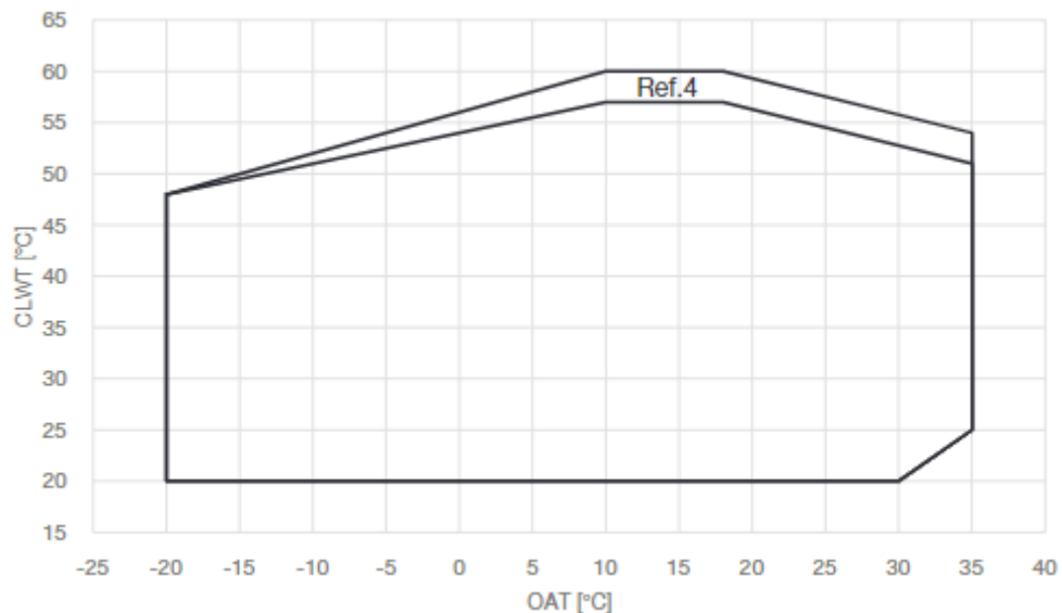
Рис. 16 - Эксплуатационные пределы для EWYTCZ в режиме нагрева
