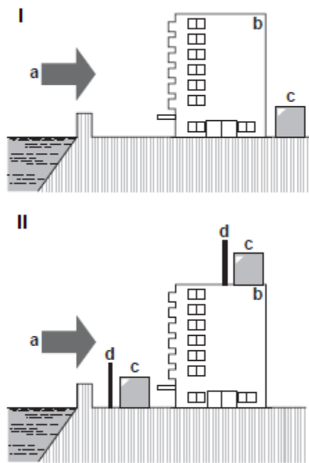
Рис. 9 –Установка наружного агрегата в прибрежной зоне
